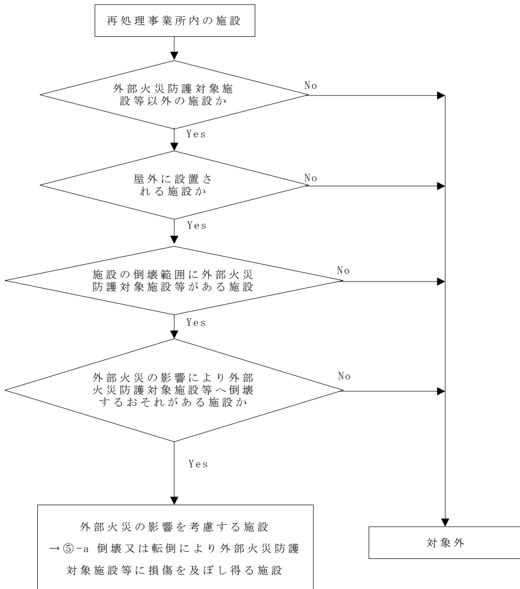
第 2-2 図 倒壊又は転倒により外部火災防護対象施設等に損傷を及ぼし得る施設の選定フロー
