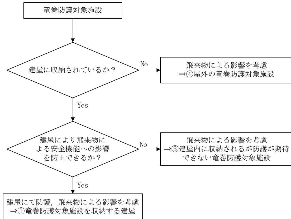
第2.1-3図 竜巻による飛来物による影響を考慮する施設の選定フロー
