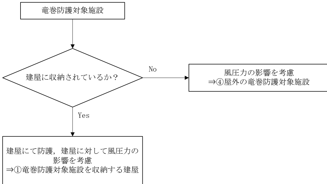
第2.1-1図 竜巻による風圧力の影響を考慮する施設の選定フロー
