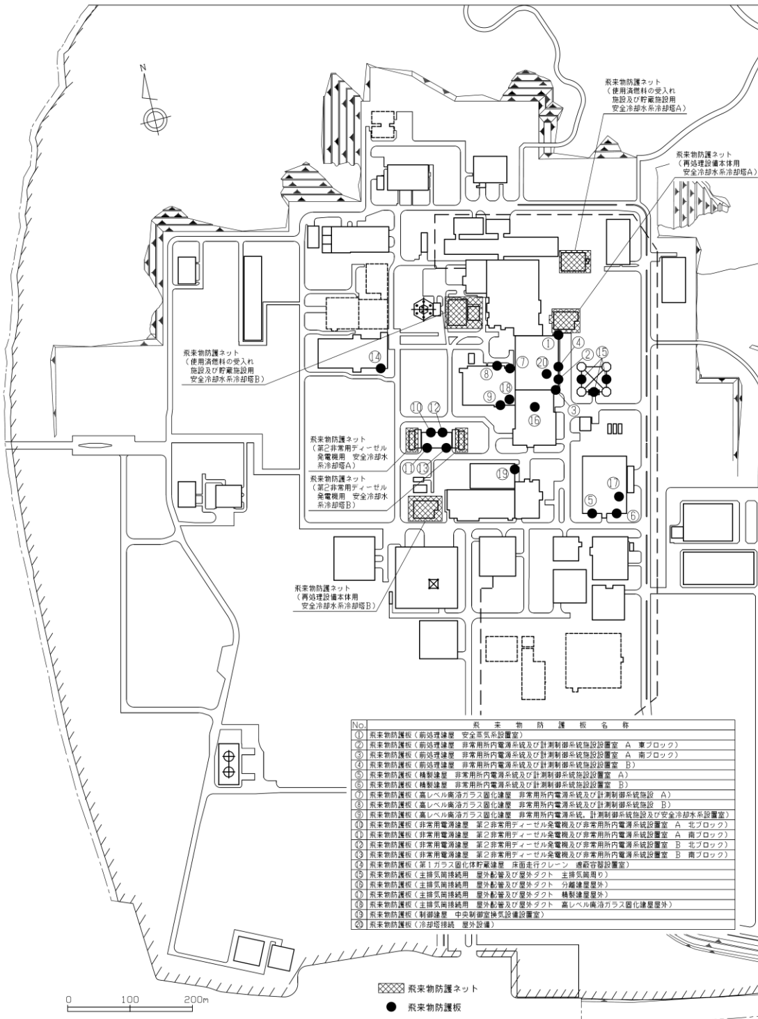
第 1.4-1 図 竜巻防護対策設備の配置
