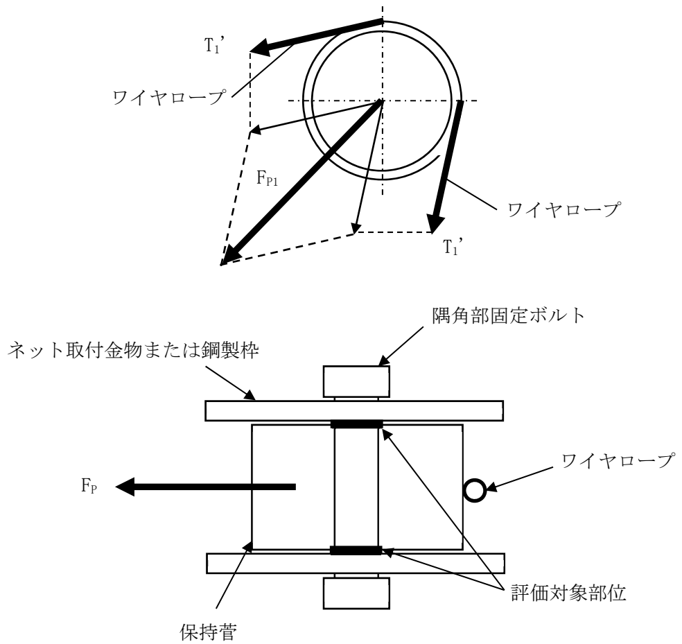
第3.5.1-4図 隅角部固定ボルトの荷重状態
