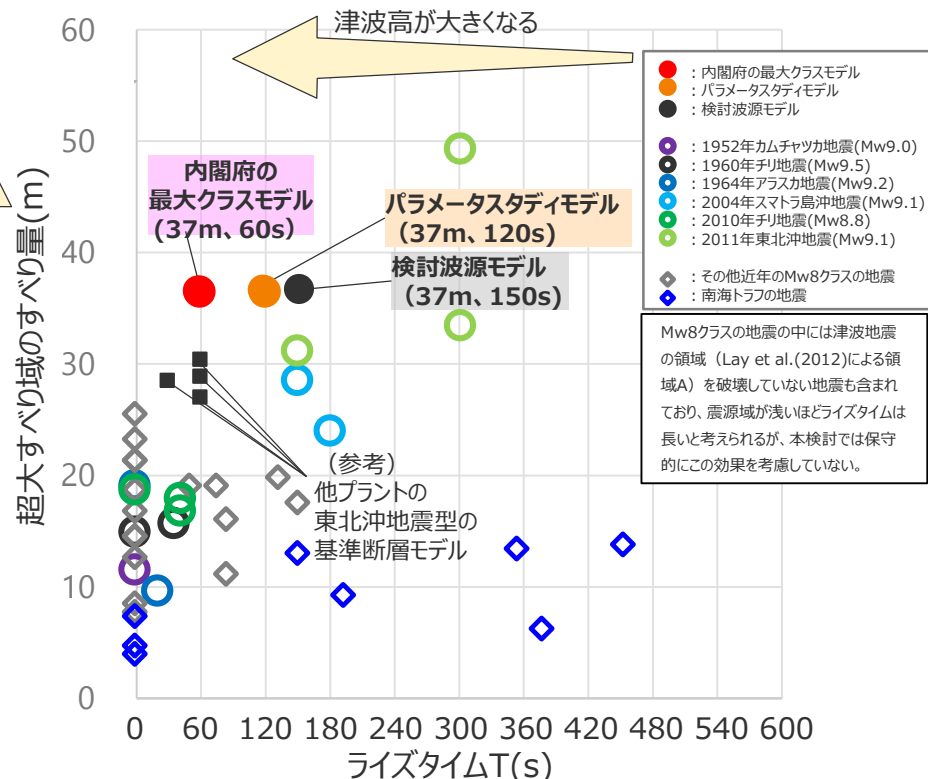
国内外の地震の津波インバージョン結果の断層すべり量とライズタイム (加藤ほか(2020)を基に作成)
