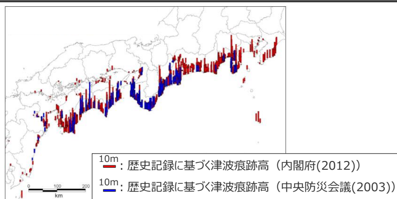
歴史記録による痕跡高の調査結果 (内閣府(2012)を基に作成)
