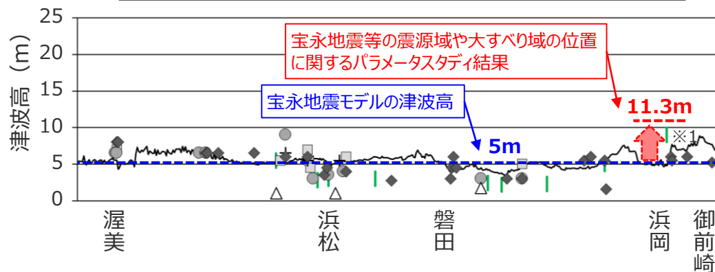
痕跡再現モデルによる海岸線の津波高と既往津波の痕跡高
