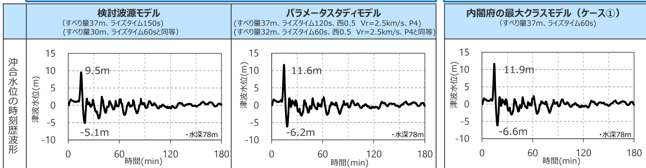
沖合10km地点の水位の比較
