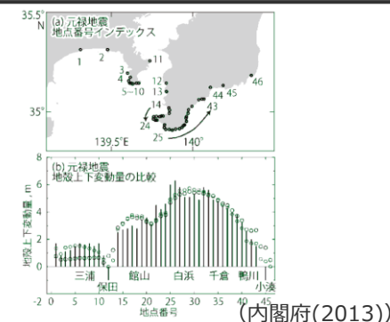
地殻変動の調査結果 (内閣府(2013))
