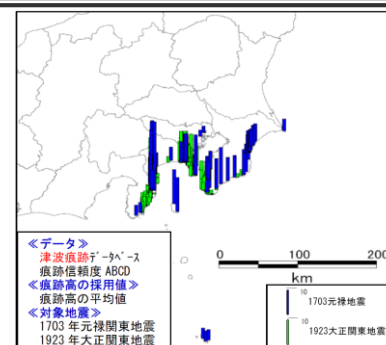
歴史記録による痕跡高の調査結果 (内閣府(2013))
