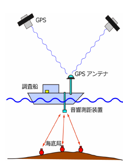
海底地殻変動観測の概要図 (中村(2010))
