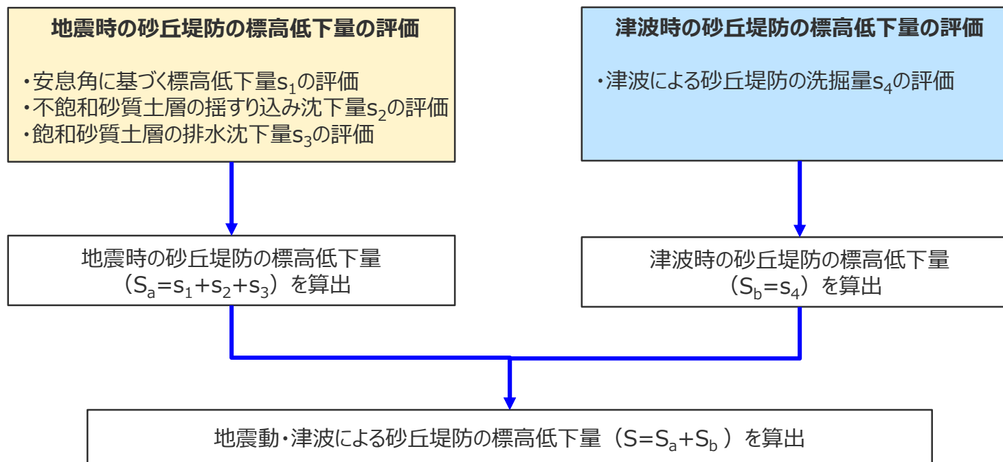
地震動・津波による砂丘堤防の標高低下の検討フロー
