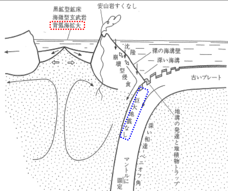
マリアナ型の沈み込み帯（上田(1989)に加筆：再掲）
