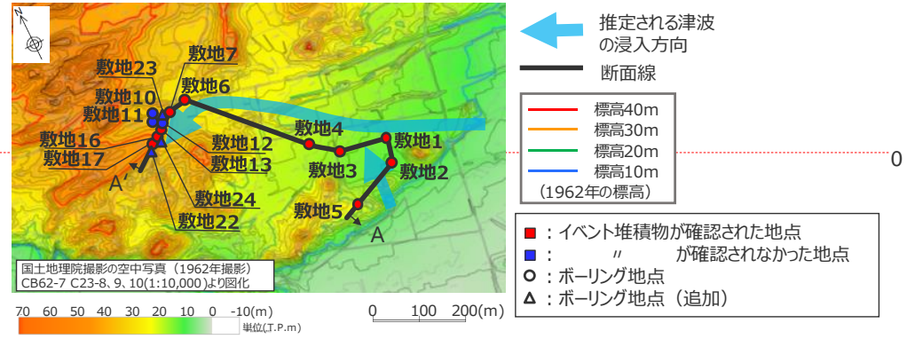
ボーリング調査地点
