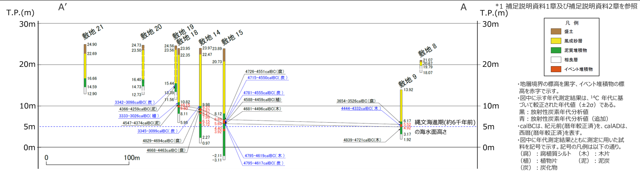
地質断面図
