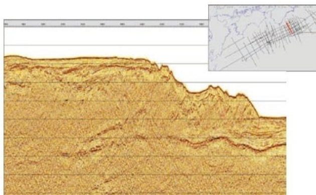
熊野灘沖
