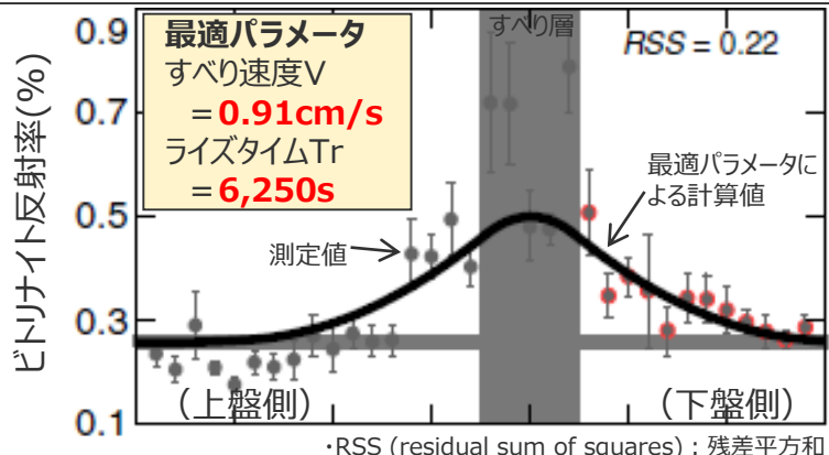
分岐断層
