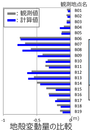
東北沖地震の痕跡高との比較 3)
