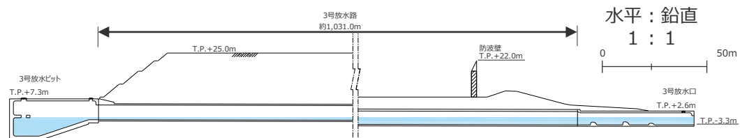
3号放水口～3号放水路～3号放水ピット縦断面図
