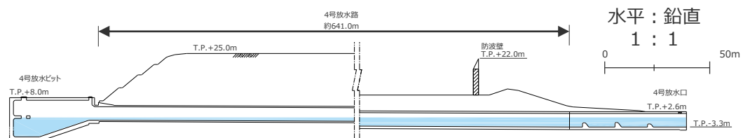
4号放水口～4号放水路～4号放水ピット縦断面図
