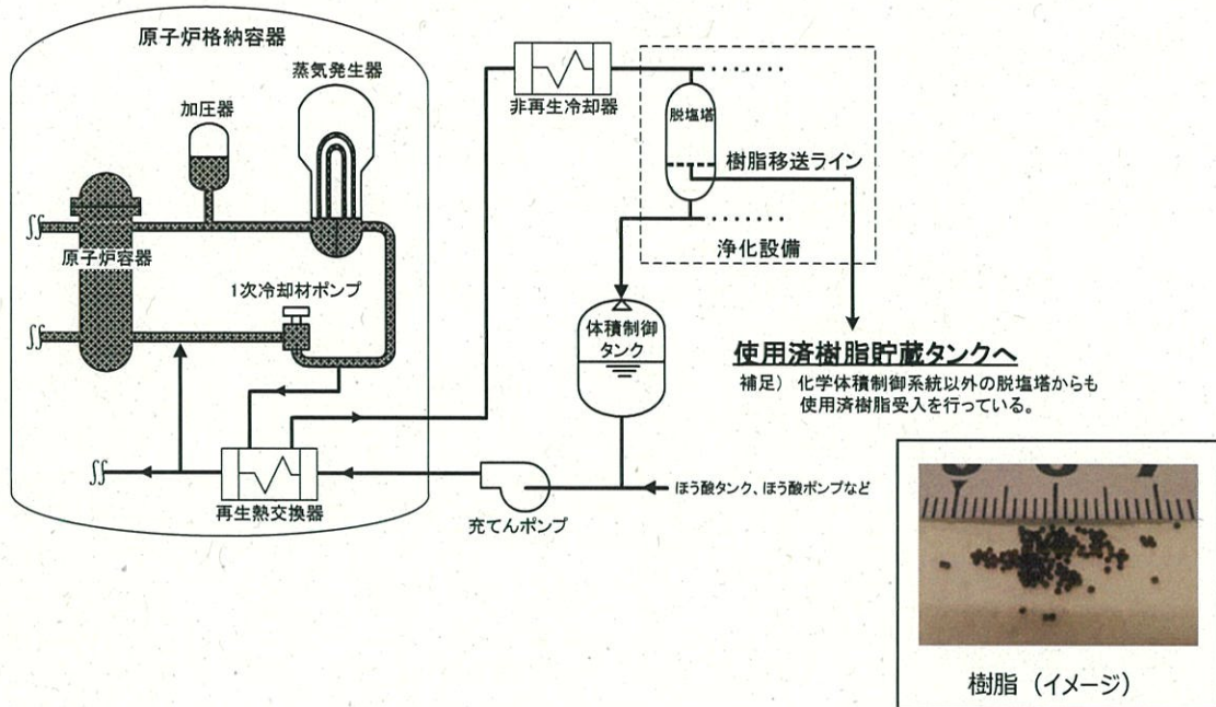
図1 化学体積制御系統(概略図)
