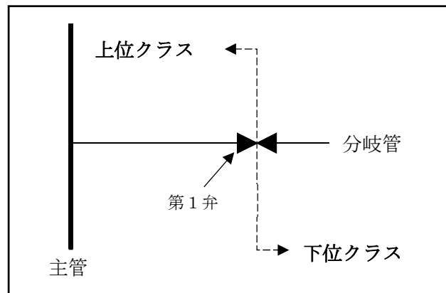
上位クラス施設との接続部例
