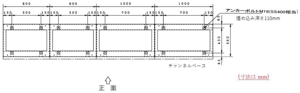
図一3 中央監視盤図
