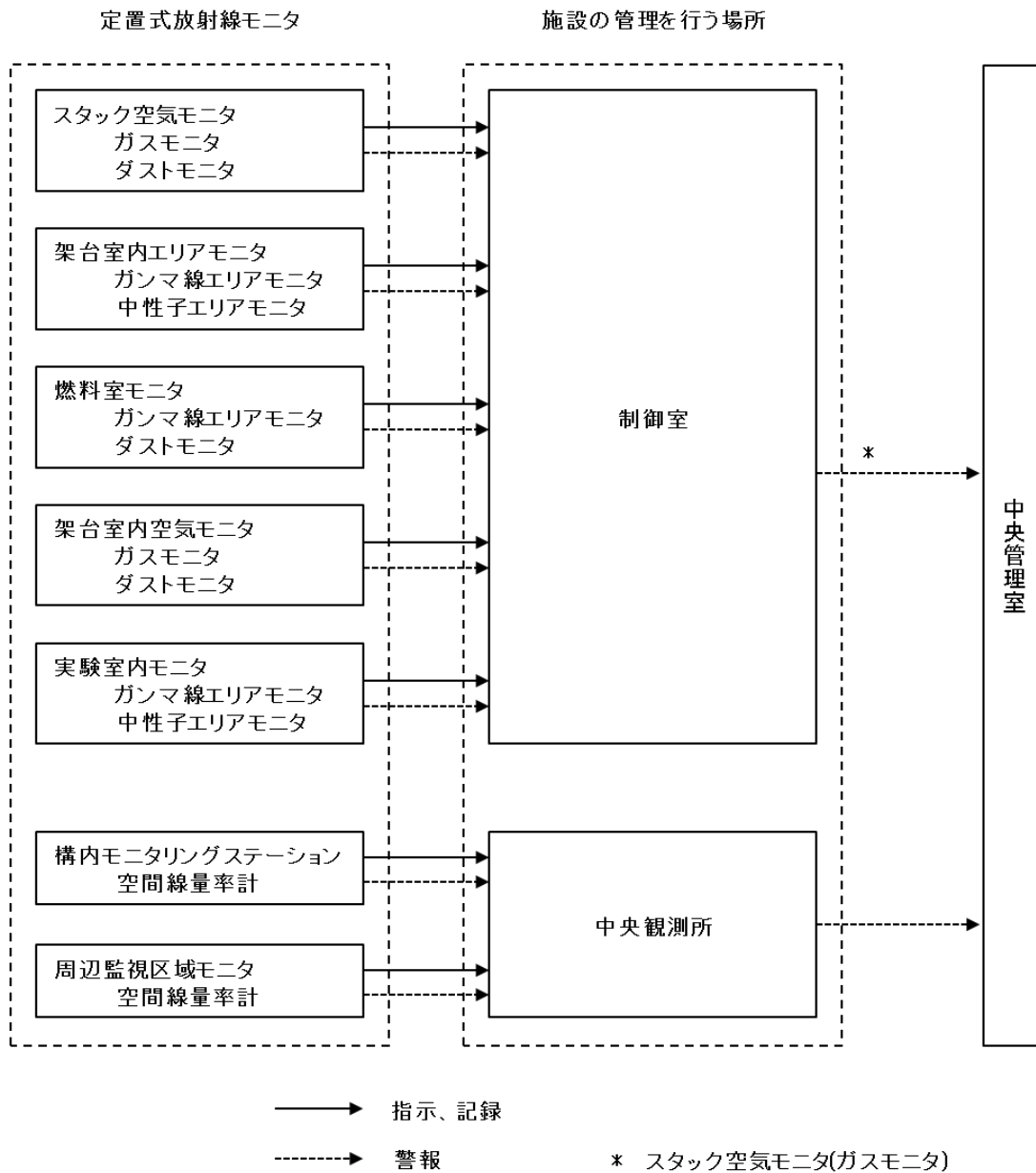
(KUCA 設置変更承認申請書)参考図 19 定置式放射線監視装置(信号及び指令系統図)
