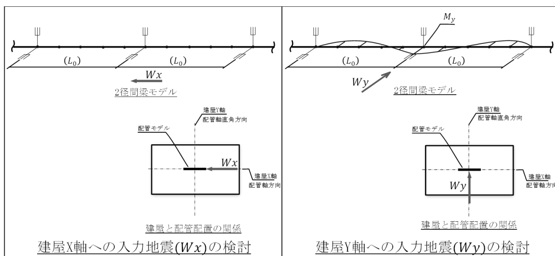
第4.5.5.1-1図 建屋X軸に沿った配管配置
