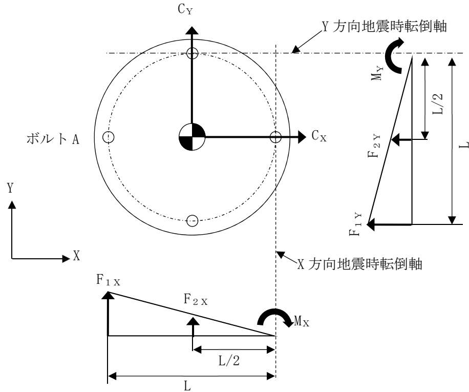
第4.5.2-3図 水平2方向の地震力による応答及び荷重イメージ
