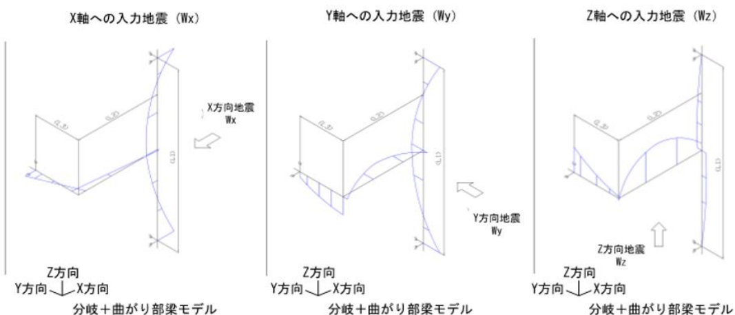
第4.5.5.1-16図(2/2) 配管(分岐+曲がり部)モデル<鉛直配管>
