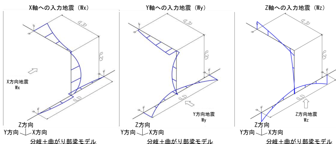
第4.5.5.1-16図(1/2) 配管(分岐+曲がり部)モデル<水平配管>
