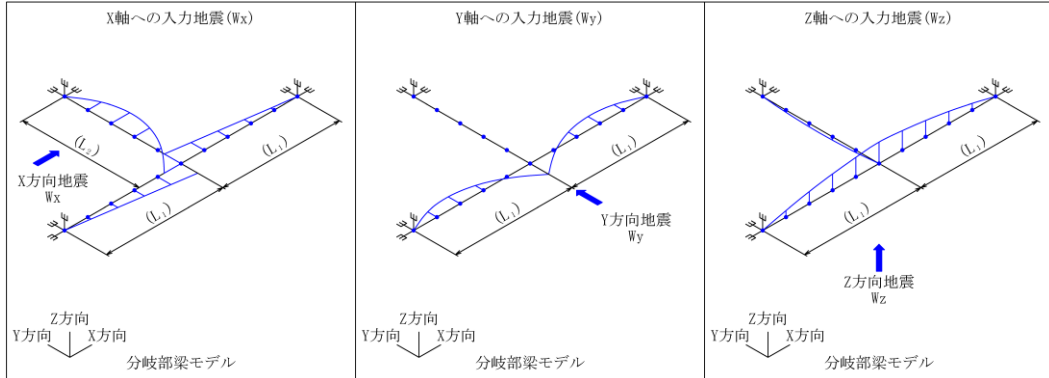
第4.5.5.1-8図(1/3) 配管(分岐部)モデル<水平配管>
