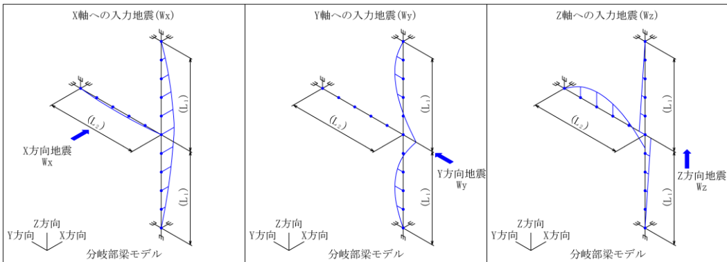
第4.5.5.1-8図(3/3) 配管(分岐部)モデル<鉛直配管(2)>
