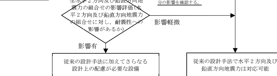
第4-1図(3/3) 水平2方向影響検討フロー(機器・配管系)
