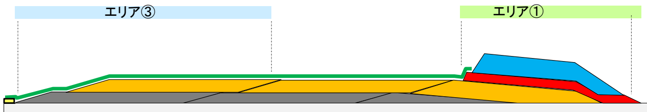
西側トレンチ工事断面
