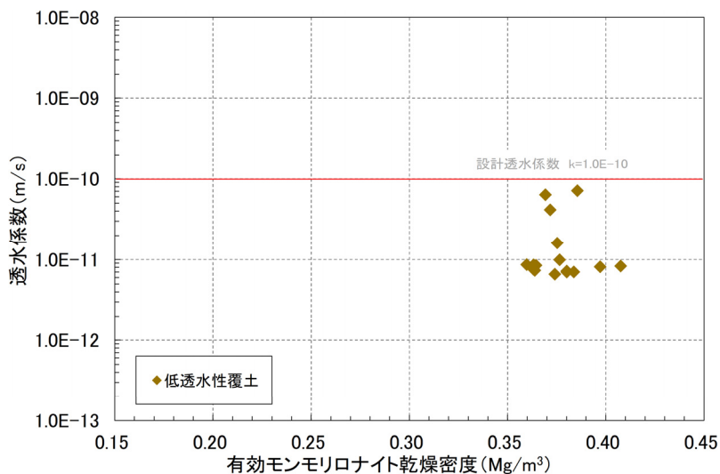
第12図 有効モンモリロナイト乾燥密度と透水係数の関係
