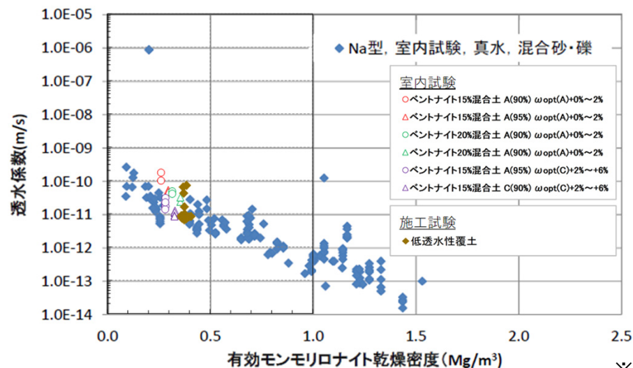
第13図 既往試験結果との比較
