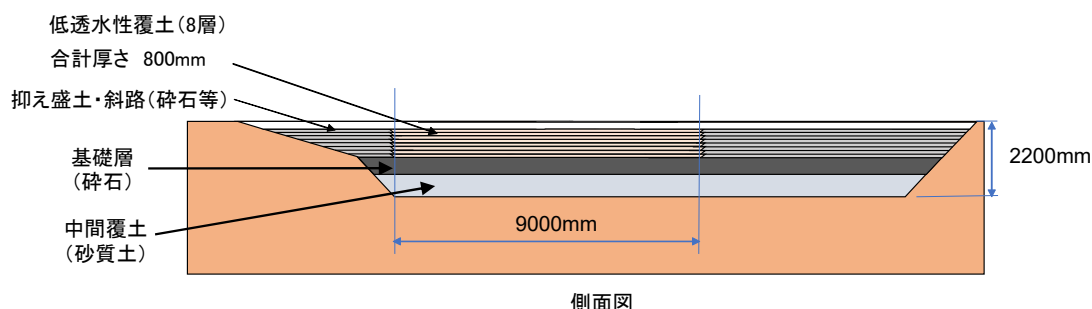
第10図 試験エリア
