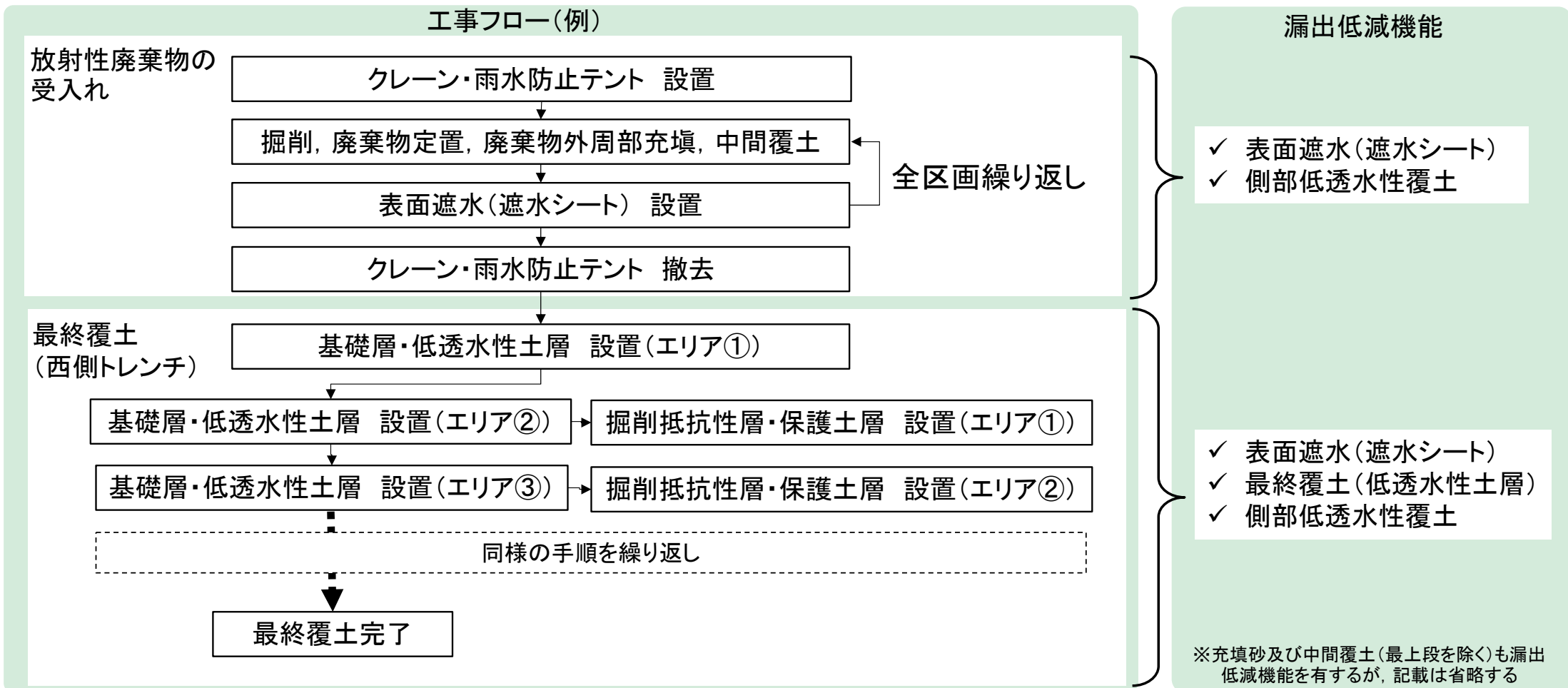
第14図 放射性廃棄物の受入れ開始から最終覆土完了までの漏出低減機能
