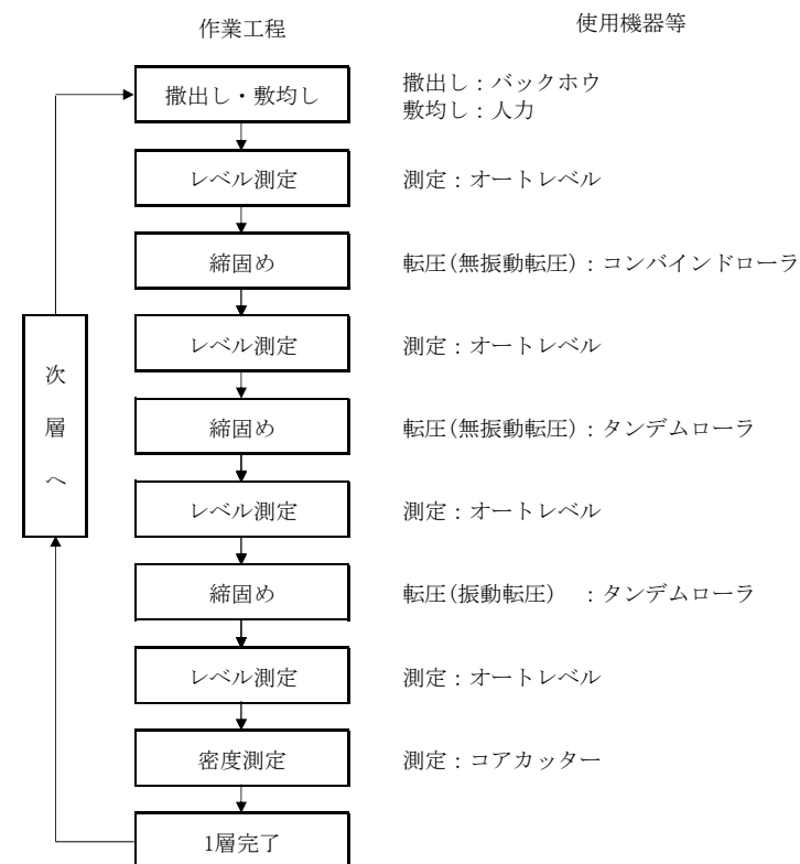
第11図 施工フロー
