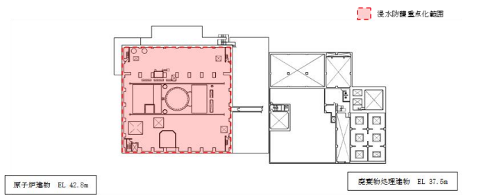
図 3-29(4) 浸水防護重点化範囲 (平面図) (4/4)
