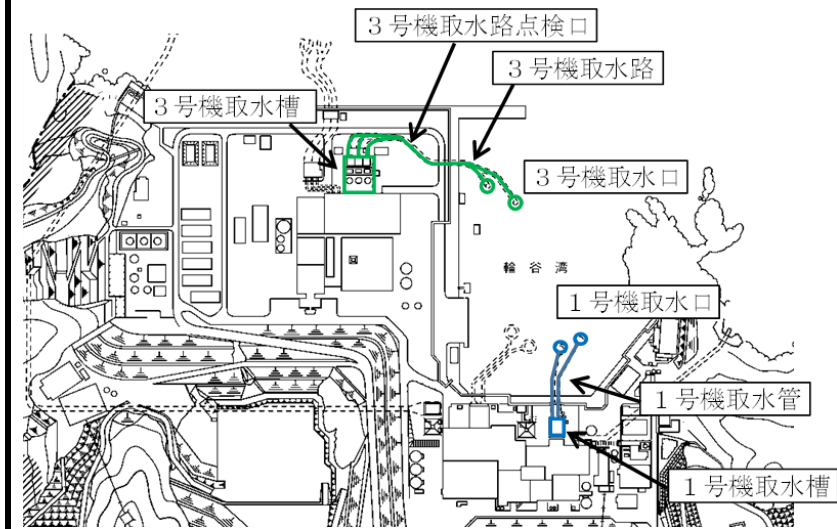
図 3-16 1, 3号機 取水施設の配置図
