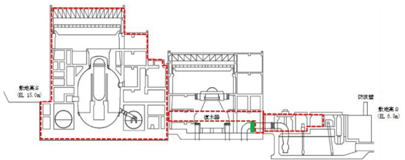
図 3-29(5) 浸水防護重点化範囲 (断面図)
