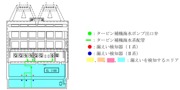
取水槽
