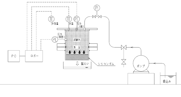
図4-6 シール材の漏えい試験の概要
