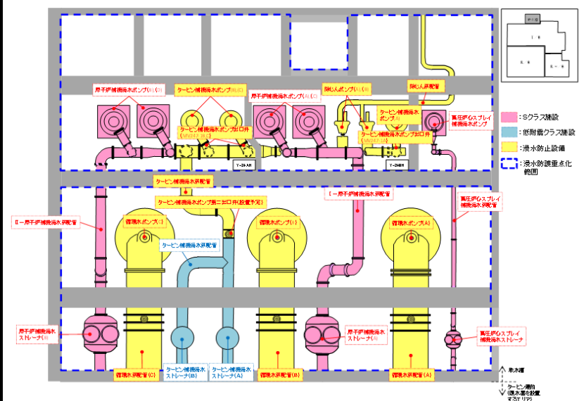
図 3-34 浸水防護重点化範囲内に設置する海域と接続する低耐震クラスの機器・配管への対策概要図 (取水槽廻り詳細図) (EL 1.1m)
