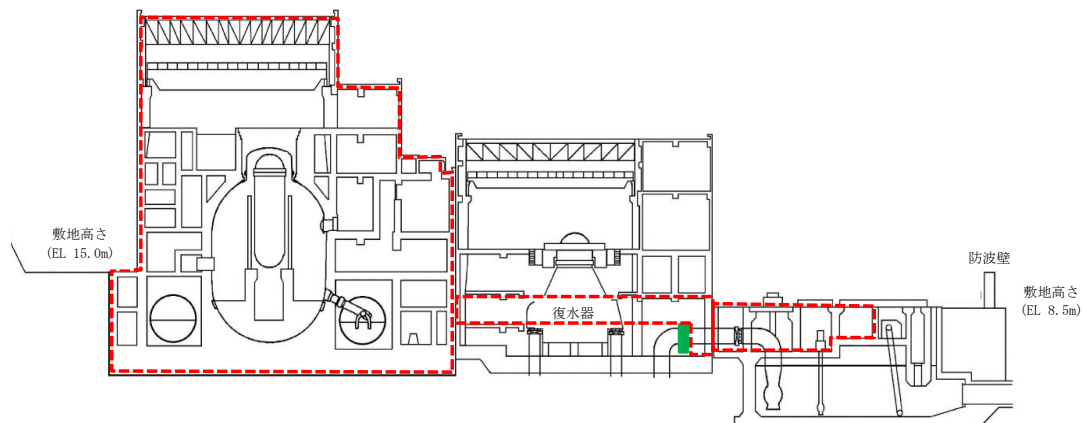
図 3-29(5) 浸水防護重点化範囲 (断面図)
