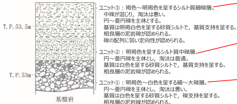
BF2地点の柱状図
