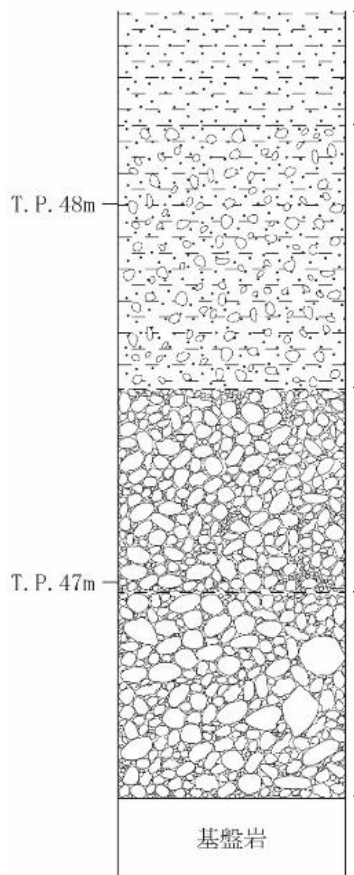
ST1地点の柱状図
