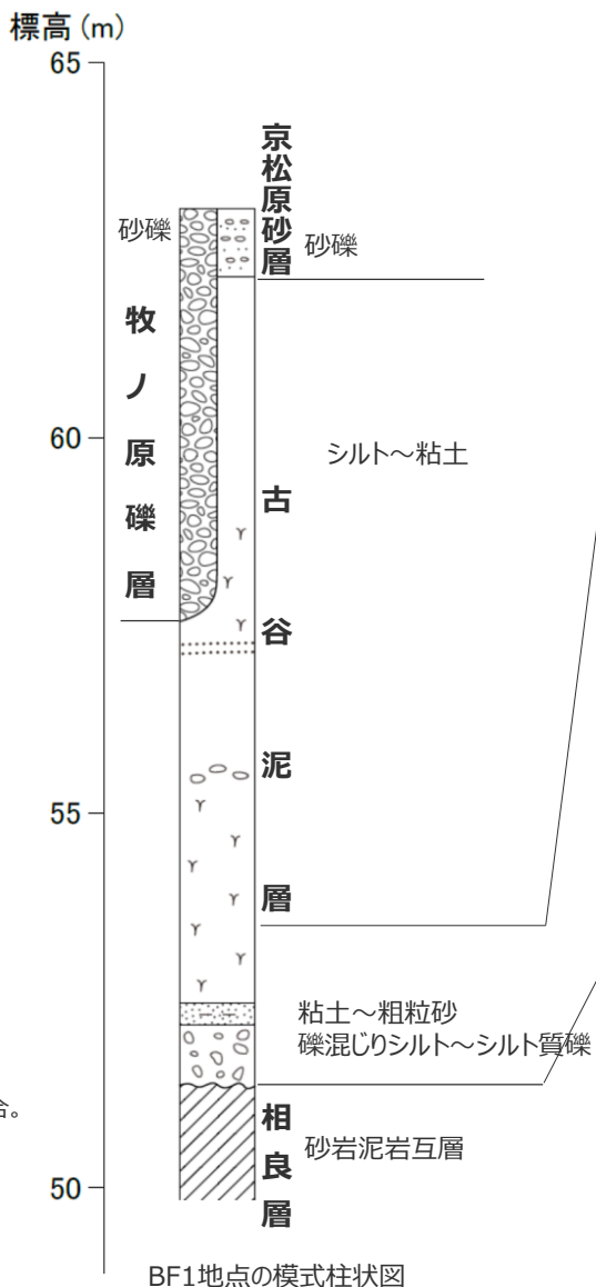
BF1地点の模式柱状図
