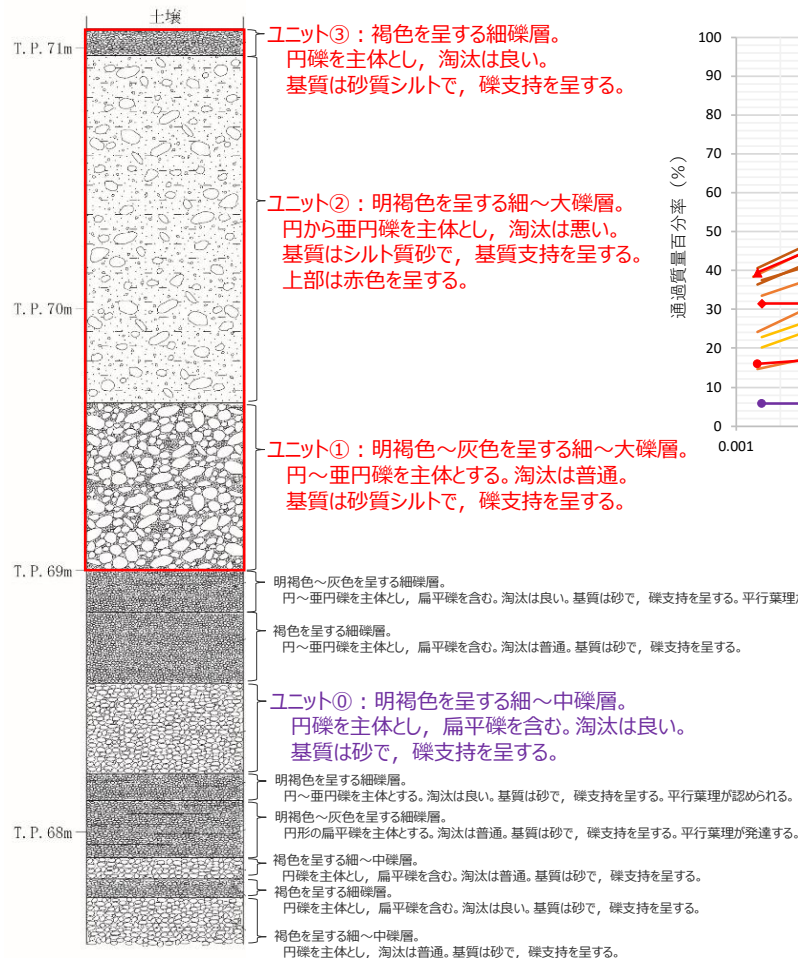
上部露頭の柱状図
