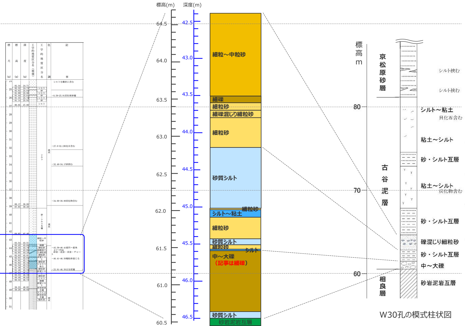
W30孔のボーリング柱状図
