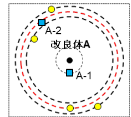
試験施工配置平面図
