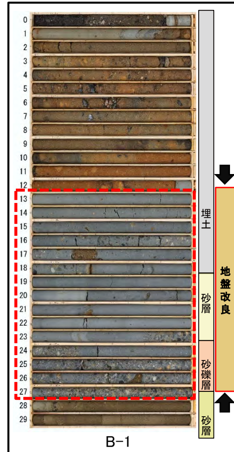
地盤改良範囲
