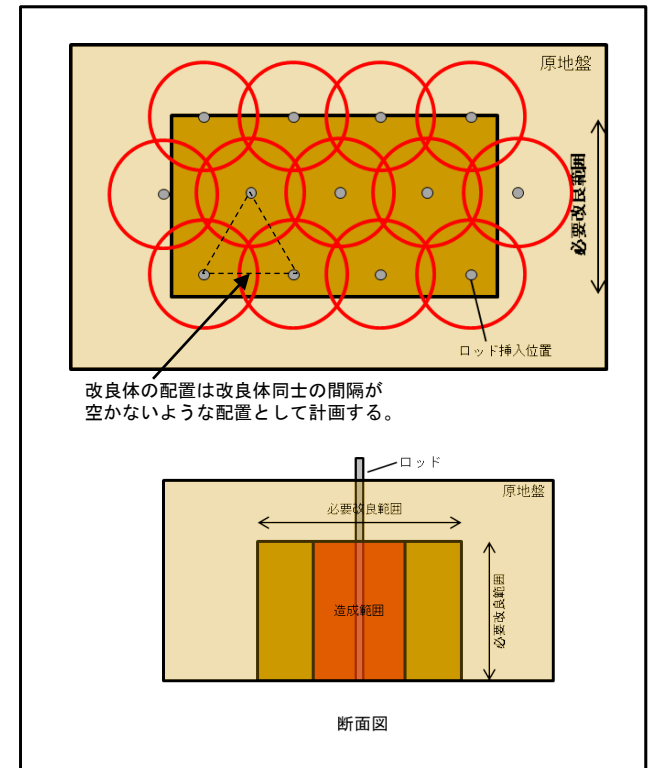
本施工での地盤改良イメージ
