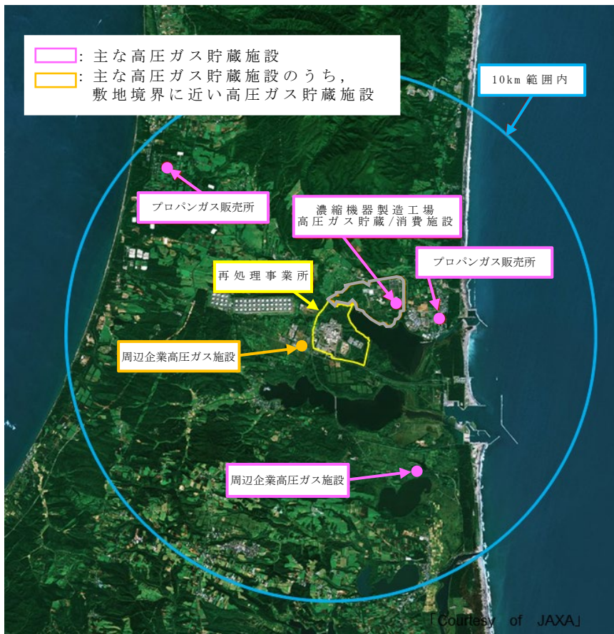
第 4-1 図 再処理事業所から 10km の範囲に存在する主な高圧ガス貯蔵施設の配置概要図
