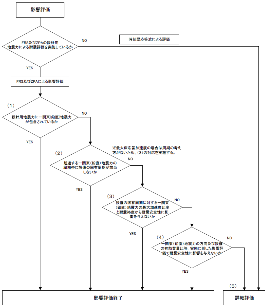
第 3-1 図 一関東評価用地震動(鉛直)の影響を考慮した影響評価対応フロー
