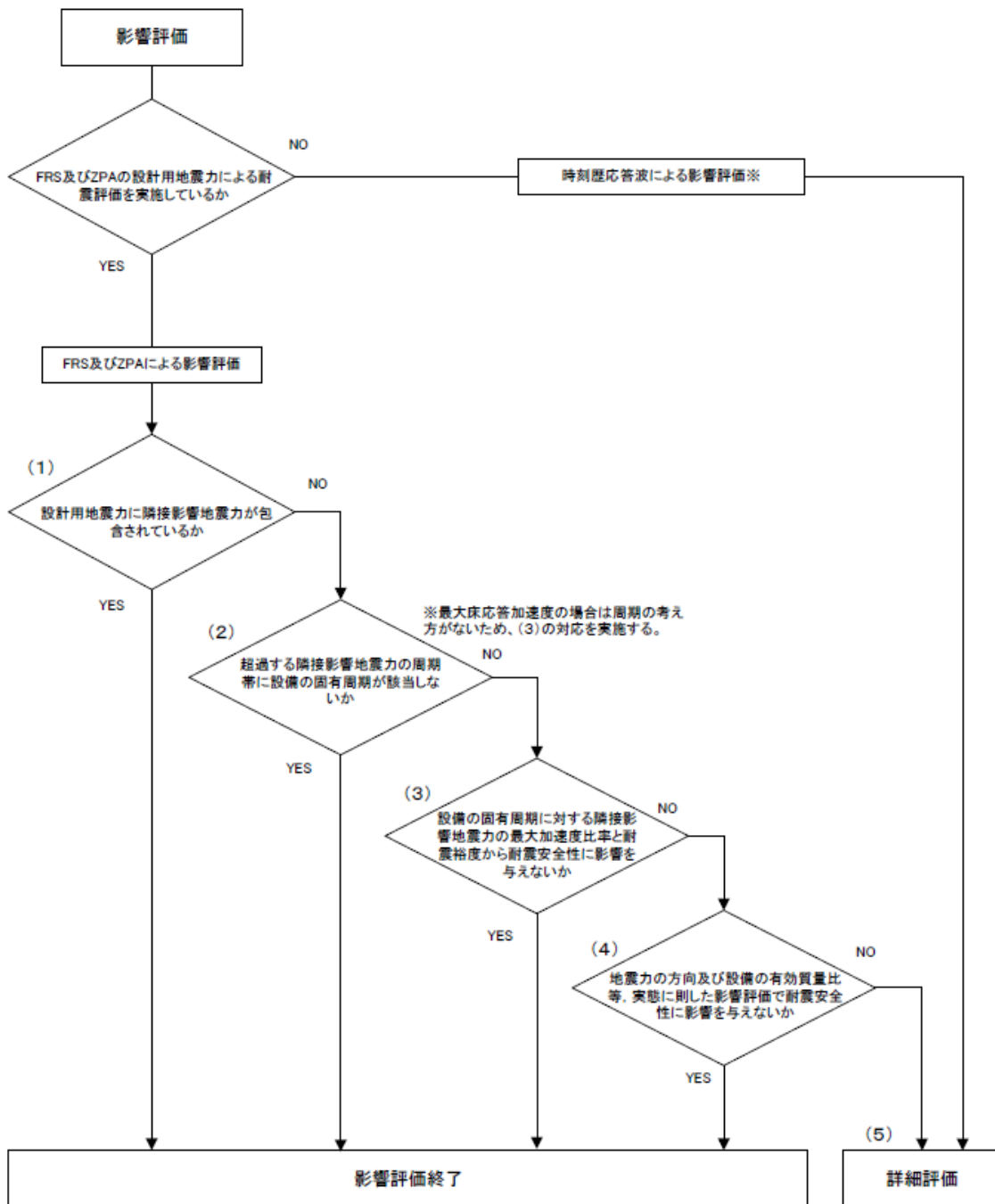
第 3.2-1 図 隣接建屋の影響を考慮した影響評価対応フロー
