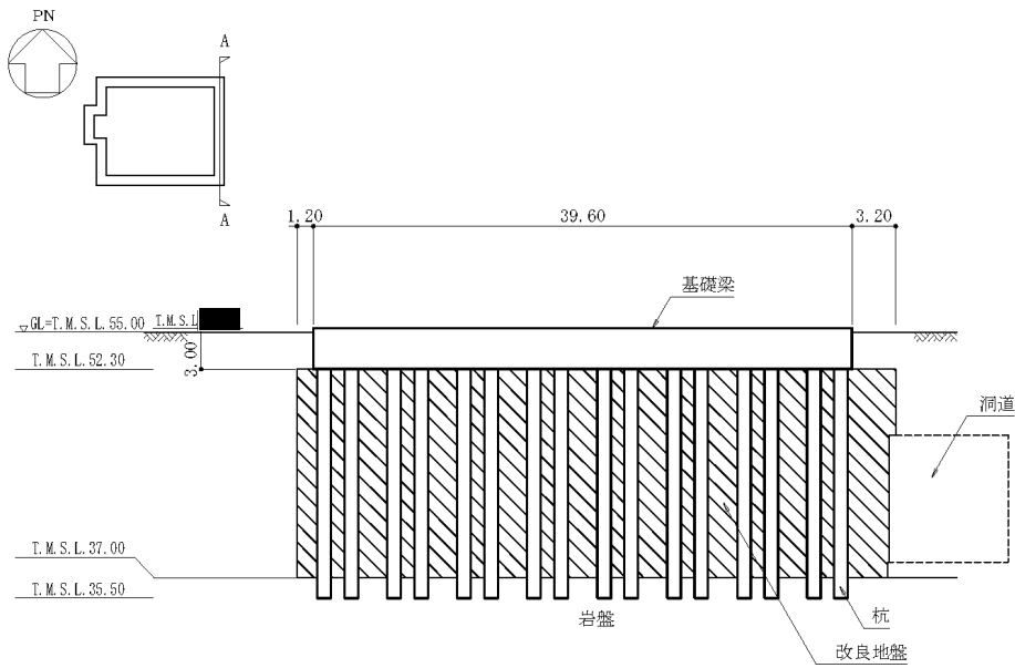
(a) A-A 断面図(NS 方向)
