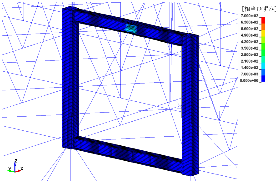
第5.3-1図 衝突位置拡大図 (飛来物防護ネットに最大ひずみが発生する時刻)
