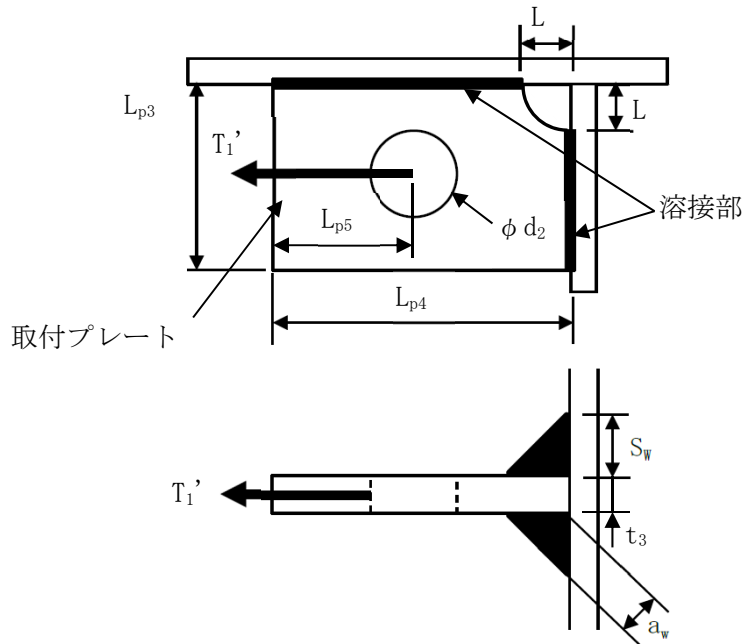
第3.5.1-5図 取付プレート(鋼製棒設置)
