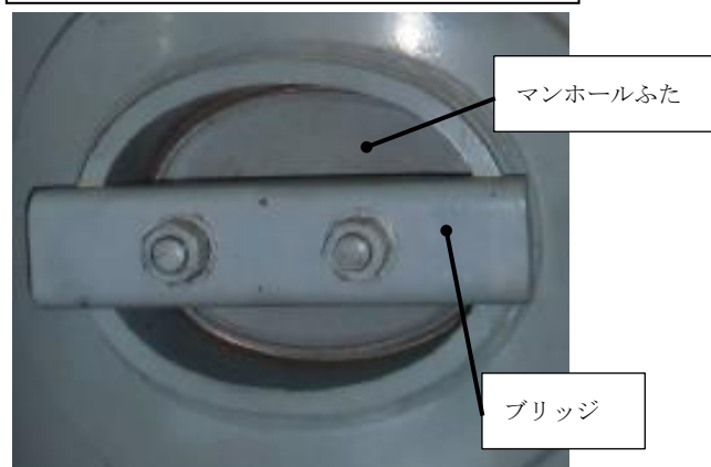
A～A矢視図 (写真)
