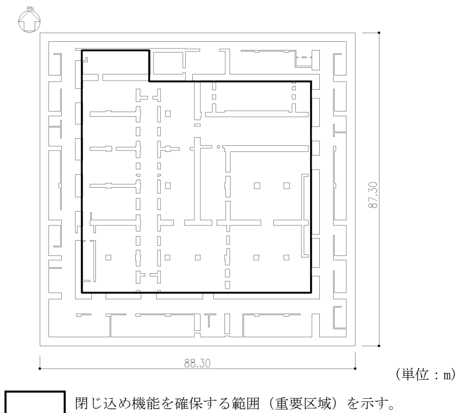
第2.2-1図 概略平面図 (T.M.S.L. 35.00m)
