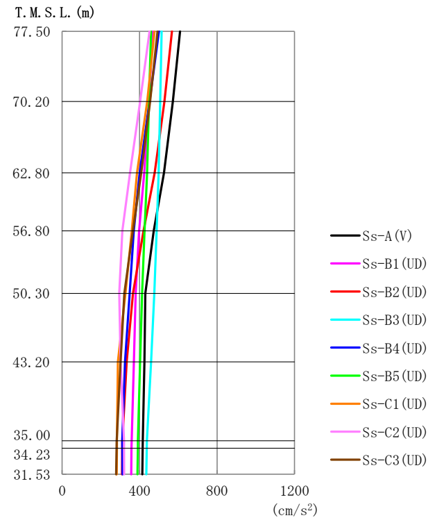
第4.1.2-9図 最大応答加速度 (基準地震動S s , ケースNo.0, 鉛直方向)
