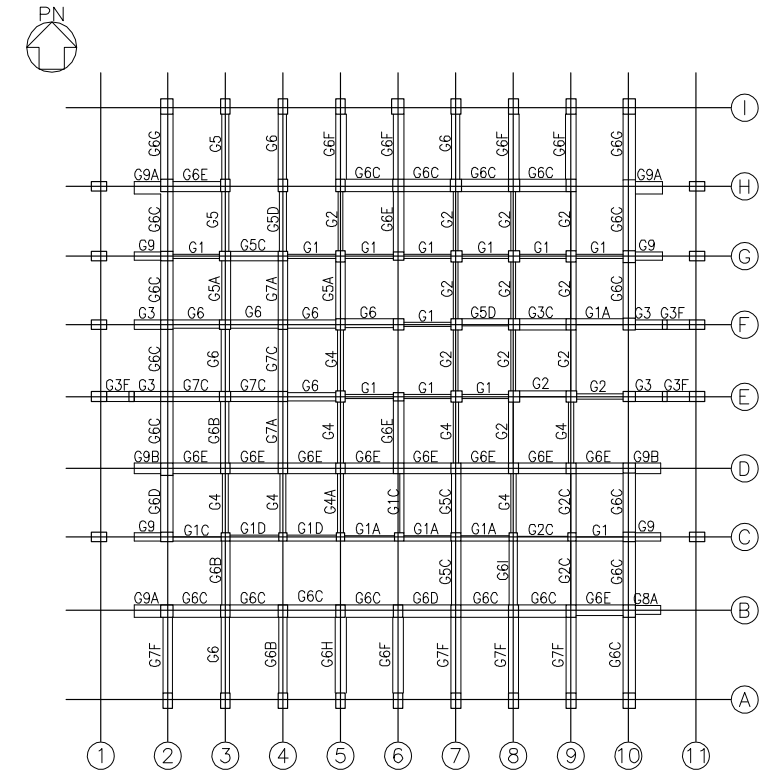
地下1階キープラン
