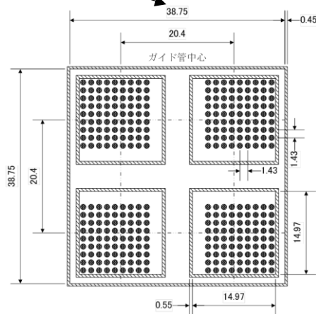
BWR燃料集合体貯蔵チャンネル (平面図)
