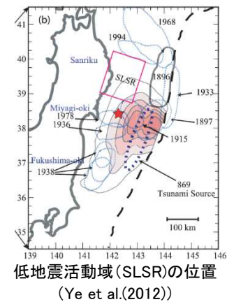
低地震活動域 (SLSR) の位置 (Ye et al.(2012))
