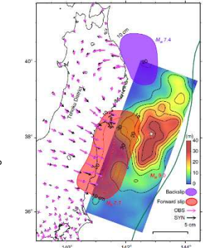
長期的なスロースリップの発生領域 (Yokota and Koketsu (2015))
