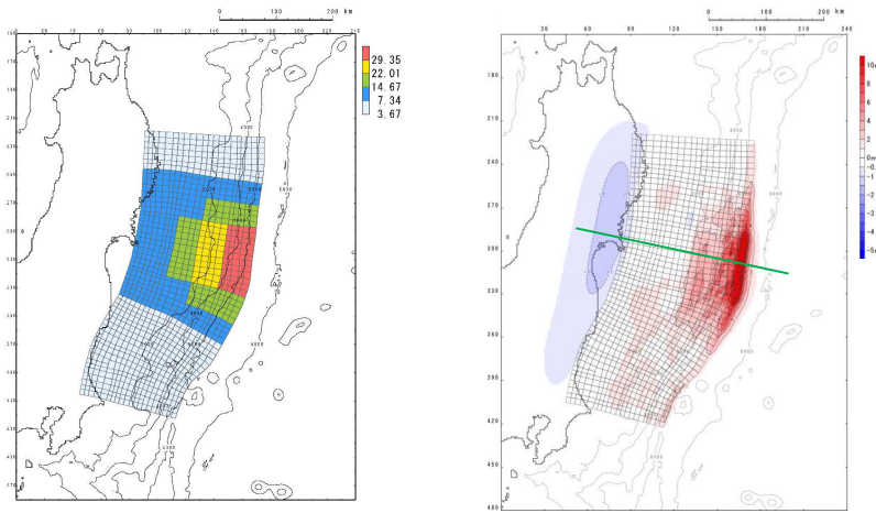
すべり量分布
