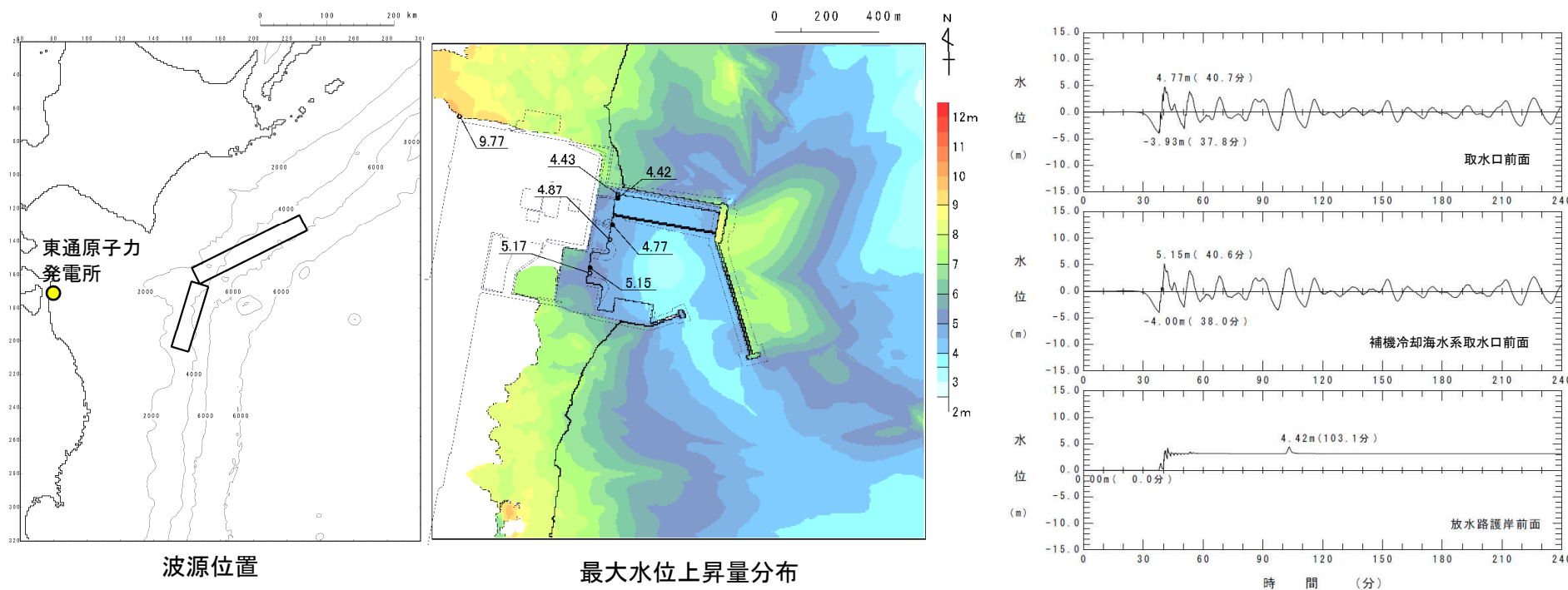
取水口前面, 補機冷却海水系取水口前面, 放水路護岸前面における水位時刻歴波形※
