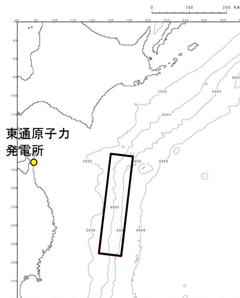
基準断層モデル (波源位置:基準)
