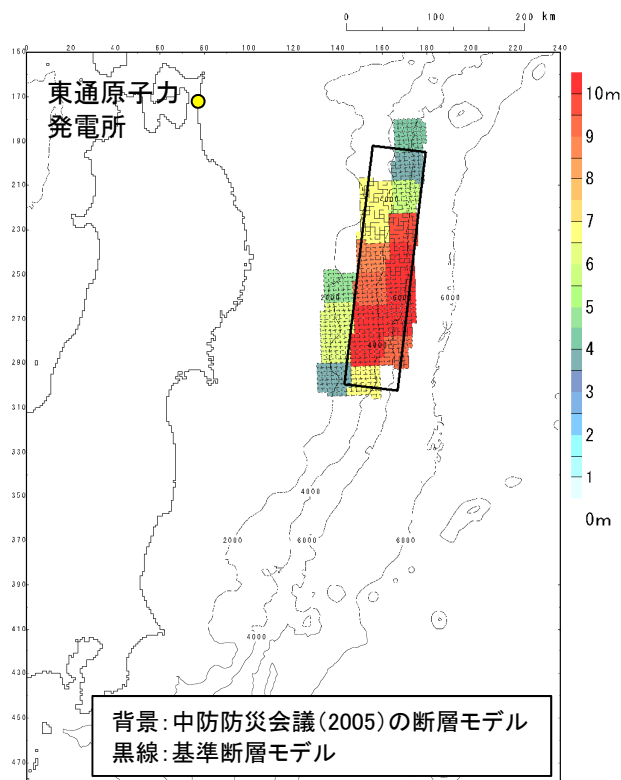
基準断層モデル (波源位置: 1896年明治三陸地震津波発生位置)
