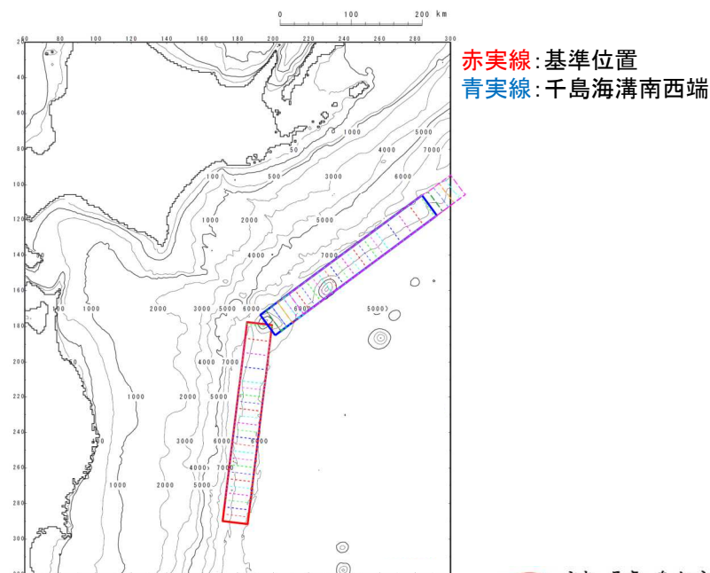
基準位置から北東へ移動の断層配置図
