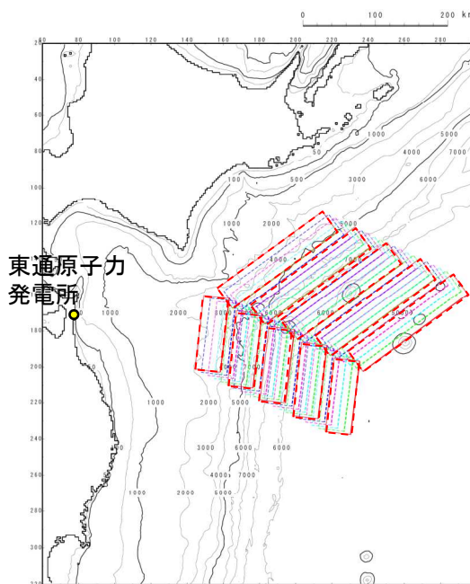
上昇側決定ケース (北東へ180km移動, 走向: 基準) 赤破線: 基準位置(中央), 50km単位移動
