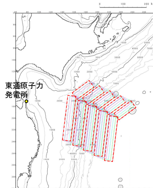
下降側決定ケース (北東へ90km移動, 走向: 基準) 赤破線: 基準位置(中央), 50km単位移動
