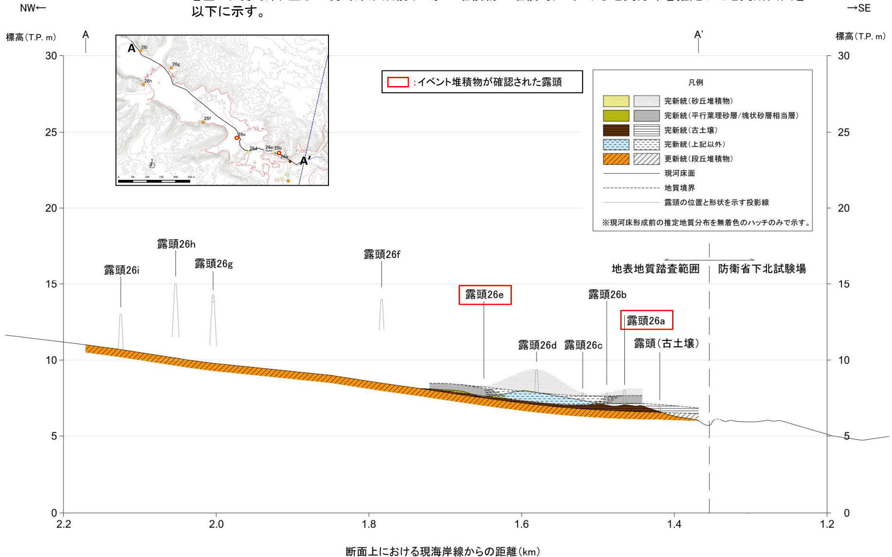
断面上における現海岸線からの距離(km) 河川に沿うAA'断面における地質断面図
