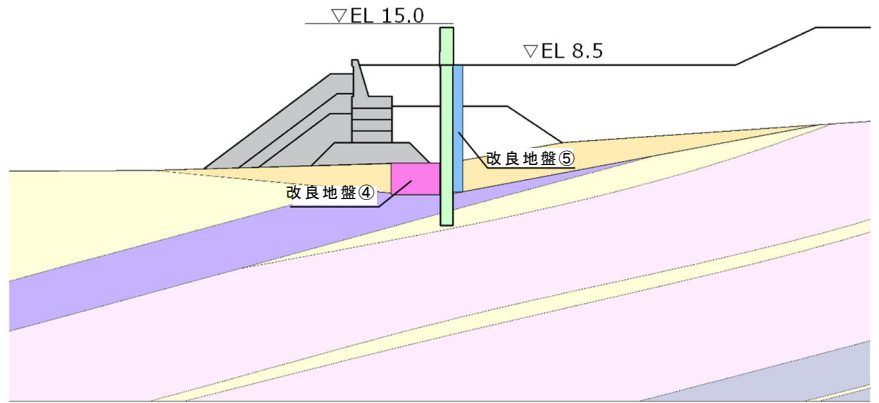
図 3-3 改良地盤の配置図 (防波壁 (多重鋼管杭式擁壁), B-B断面)
