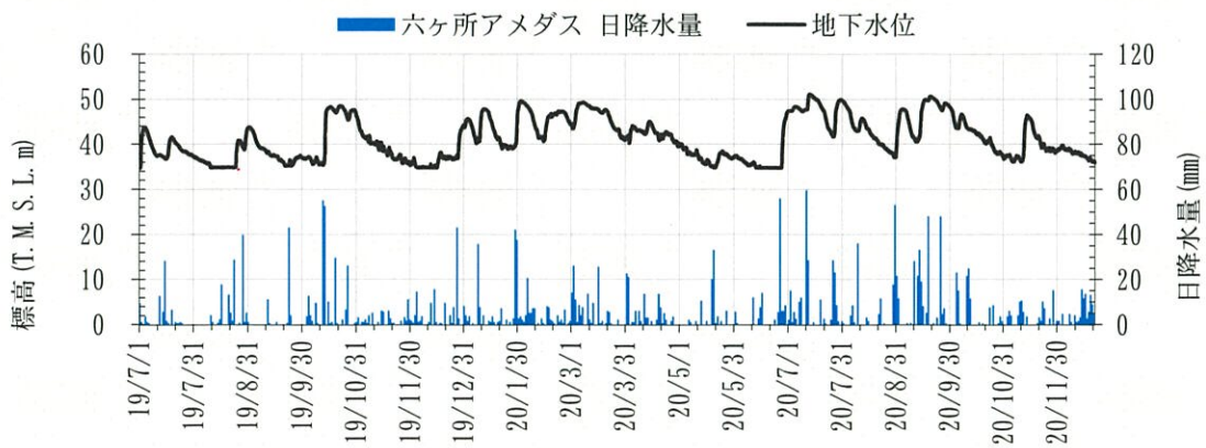
第 1. -1 図 (15) ARW-2 孔における地下水水位観測記録と降水量データ
