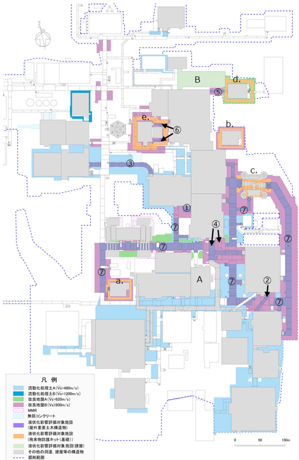
第 5.1-1 図 液状化影響評価対象施設の位置
