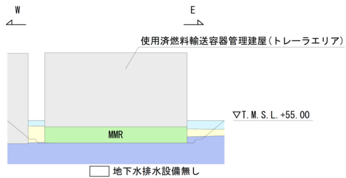
B - B 立面図
