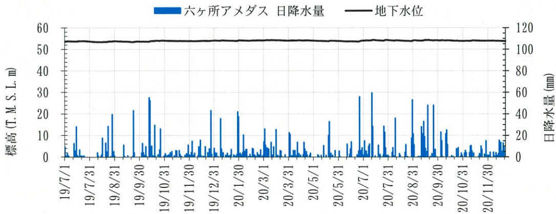
第 1. -1 図 (1) KD-3 孔における地下水水位観測記録と降水量データ
