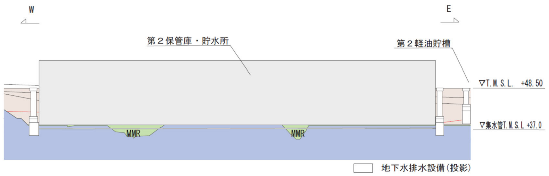
B - B 立面図
