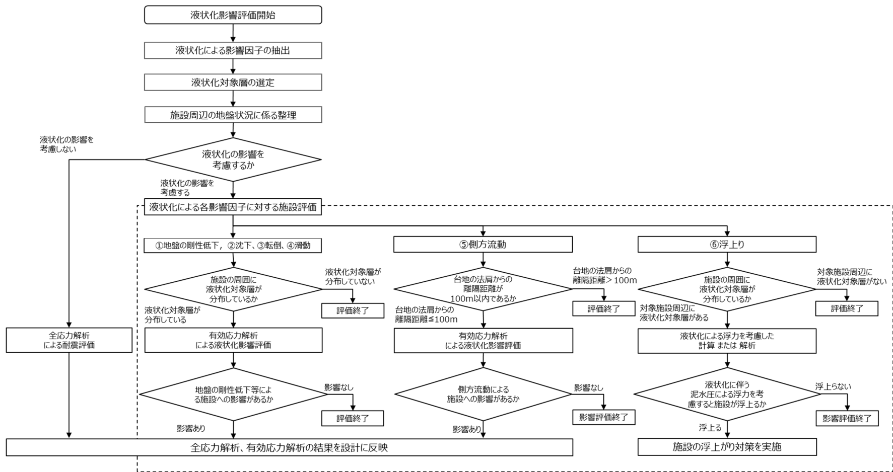
第 5.1-2 図 液状化影響評価フロー
