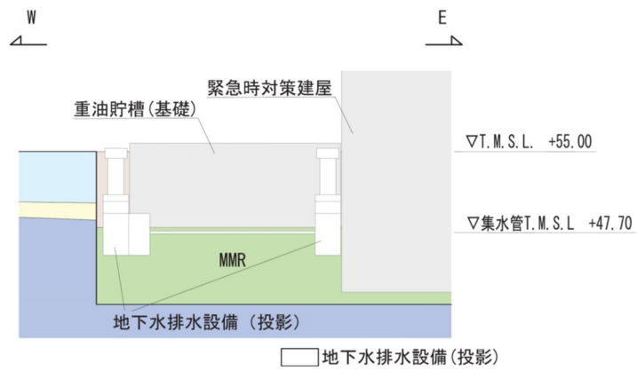
B - B 立面図
