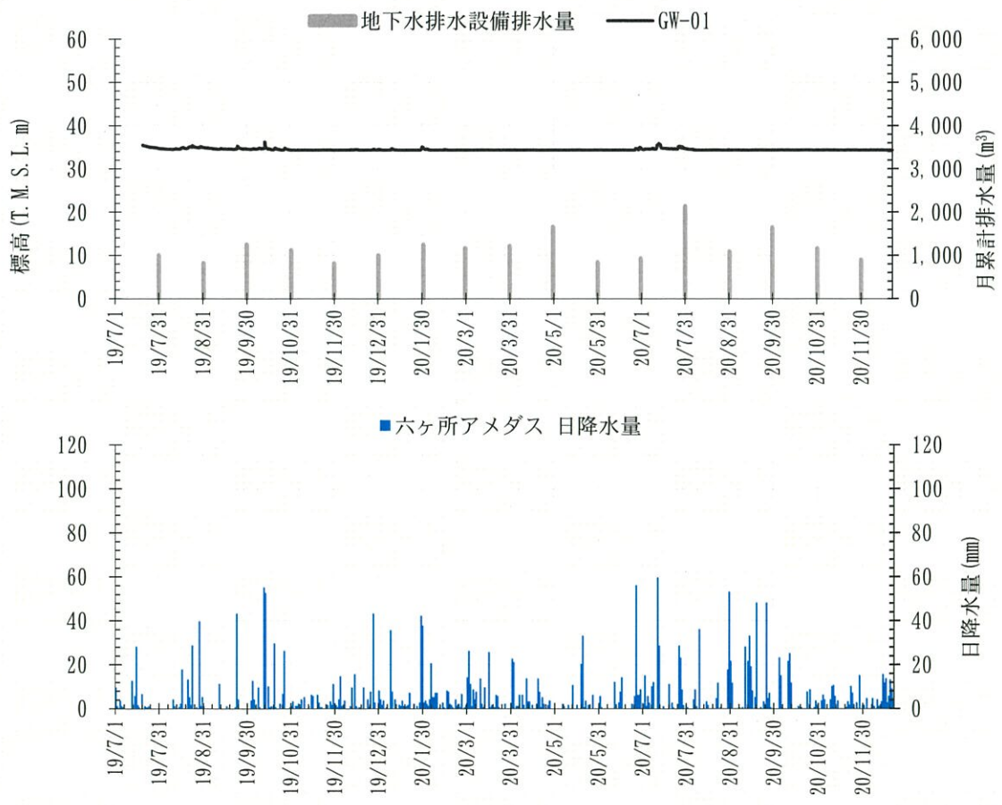
第 1. -3 図 (1) 地下水排水設備による排水量とその近傍の地下水位及び日降水量の比較
