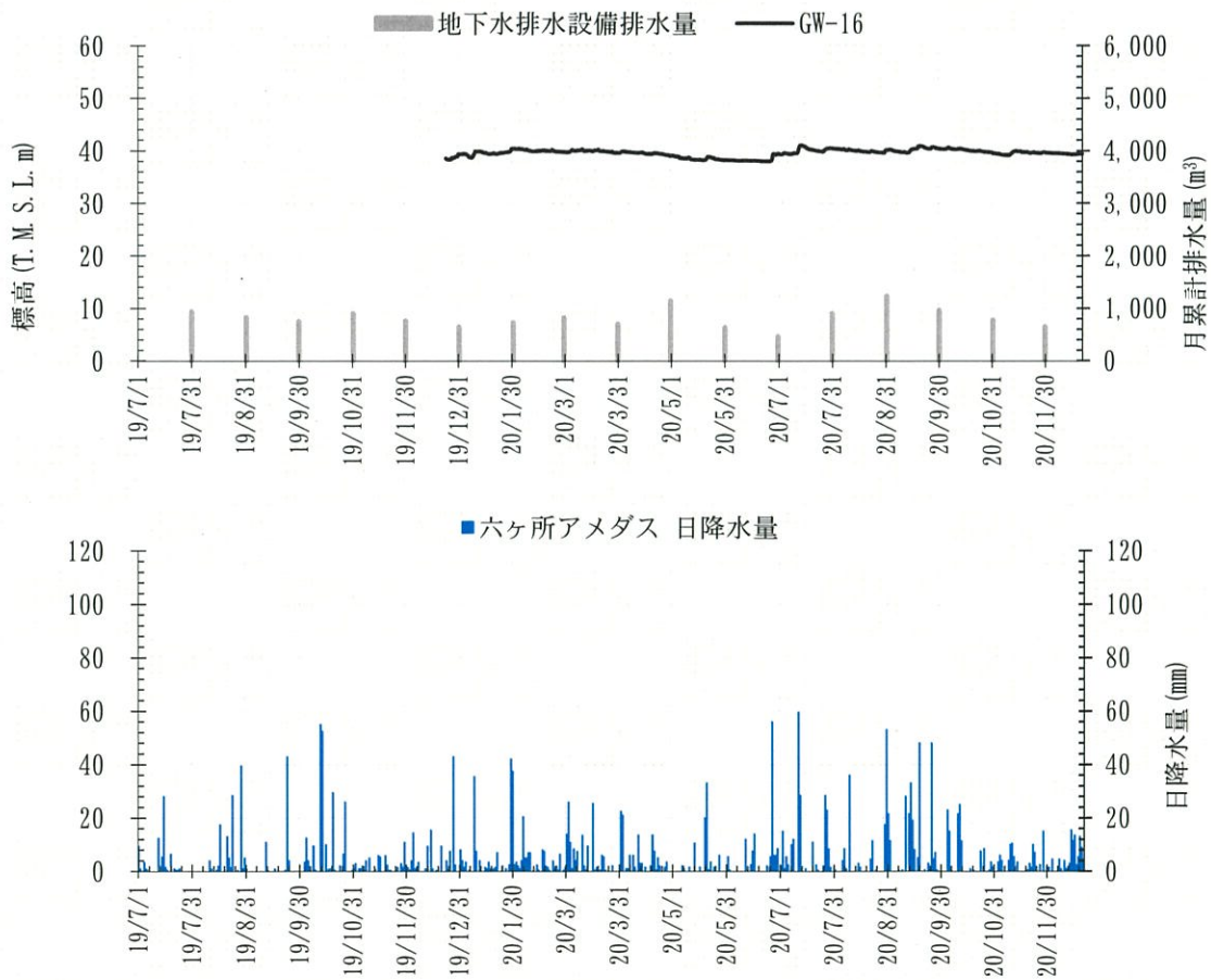
第 1. -3 図 (5) 地下水排水設備による排水量とその近傍の地下水位及び日降水量の比較
