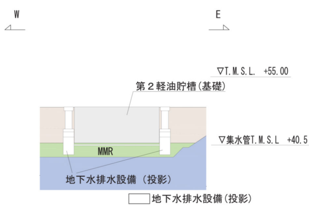
B - B 立面図
