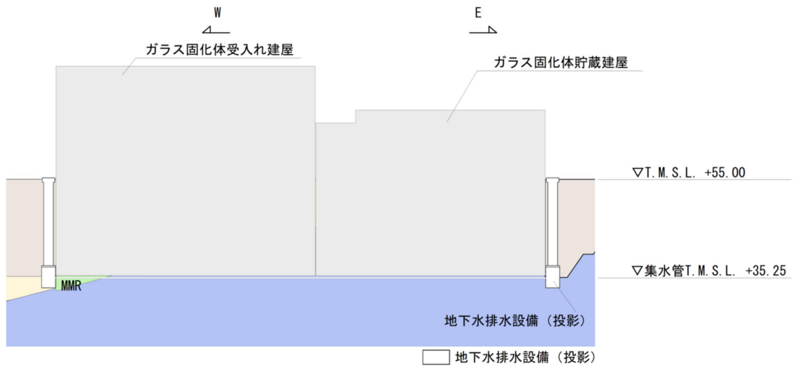
B - B 立面図
