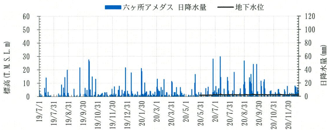
第 1. -1 図 (18) AR-4 孔における地下水位観測記録と降水量データ
