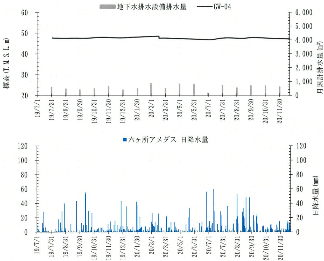
第 1.-3 図(2) 地下水排水設備による排水量とその近傍の地下水位及び日降水量の比較
