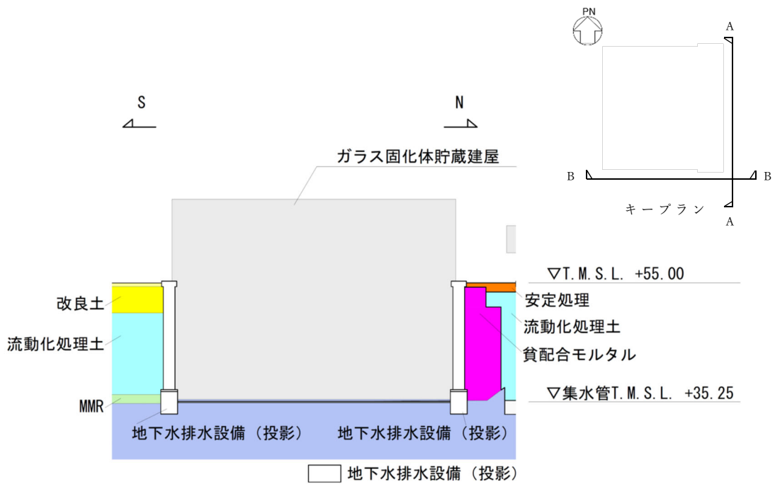
A - A 立面図
