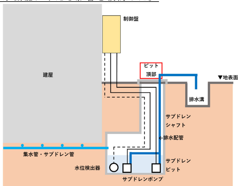
第 1-1 図 地下水排水設備概要図
