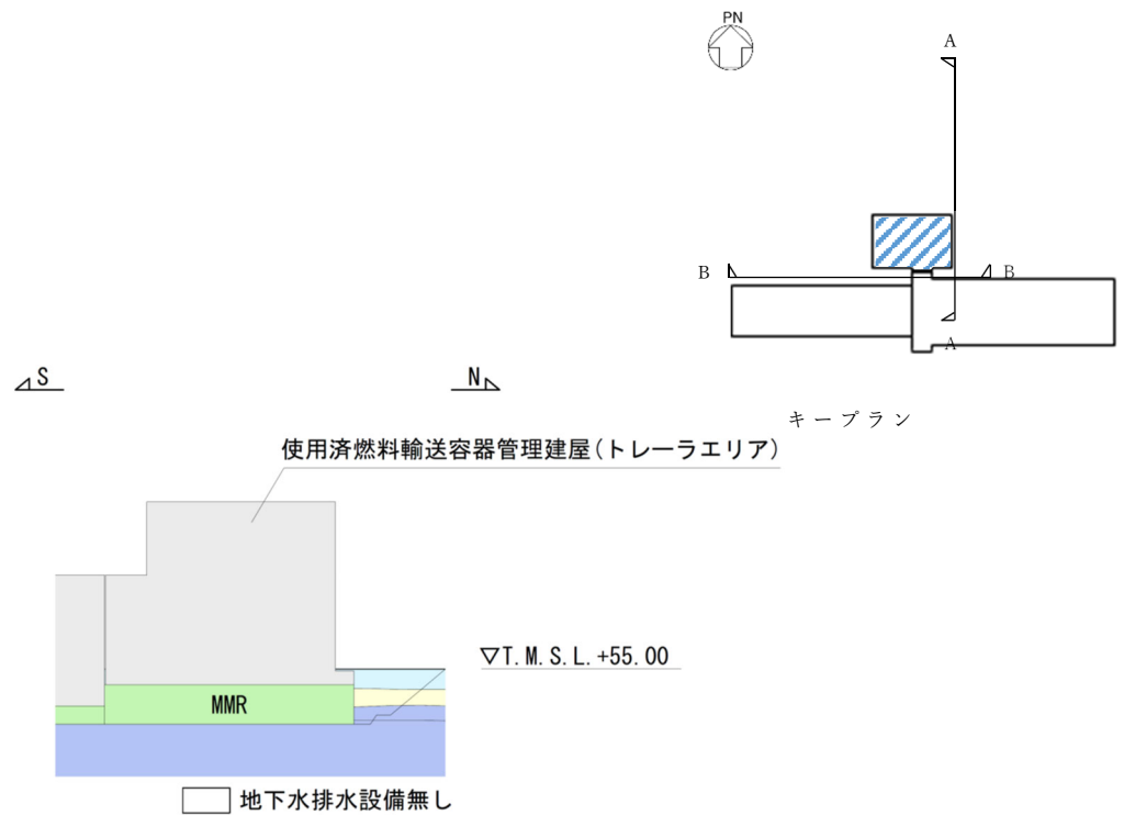
A - A 立面図
