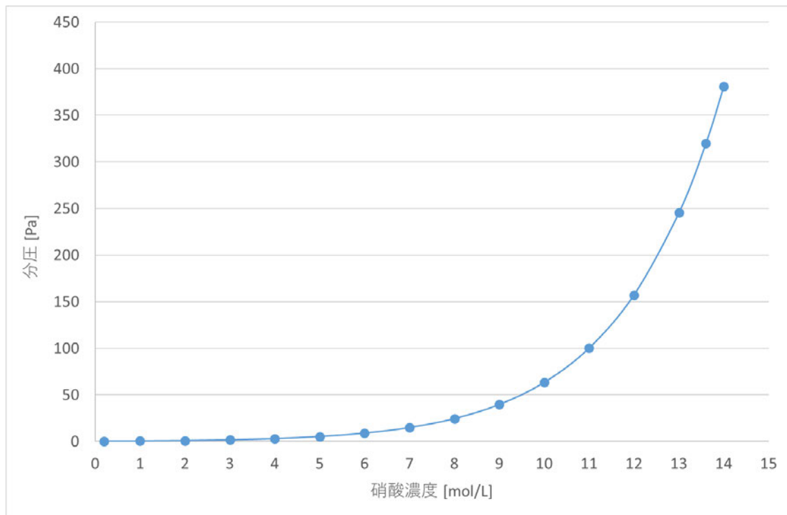
第4図 温度30°Cにおける硝酸濃度の違いによる分圧の変化
