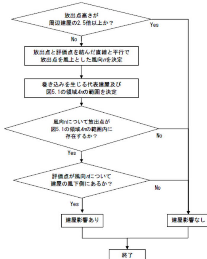
第2図 建屋影響有無の判断基準（被ばく評価手法（内規）の図5.2より）
