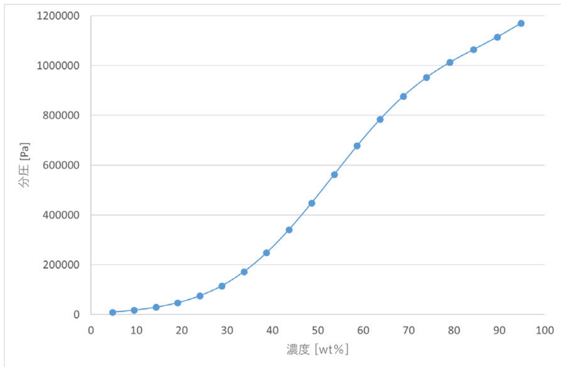
第5図 温度約32.2°Cにおけるアンモニア濃度の違いによる分圧の変化
