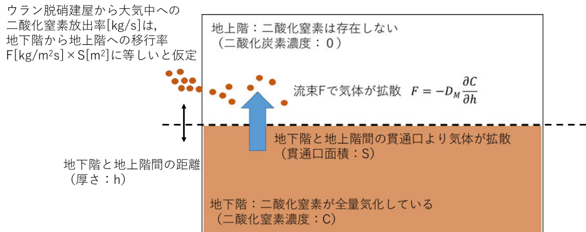
第7図 ウラン脱硝建屋における放出率評価の概念図
