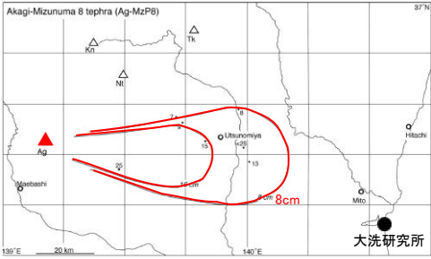
第22図 赤城水沼8テフラ(Ag-MzP8)の分布 数字は降下火砕堆積物の層厚で、単位はcm。Ag = 赤城火山；Hu = 燧ヶ岳火山；Kn = 鬼怒沼火山；Ni = 男体火山；Tk = 高原火山。
