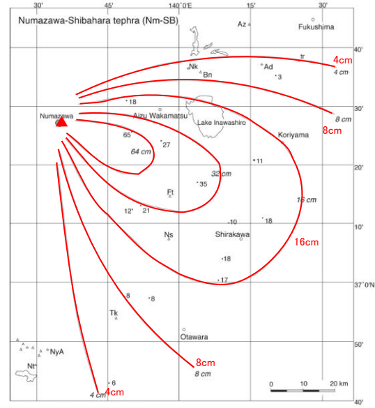
第28図 沼沢芝原テフラ (Nm-SB) の分布。 数字は降下火砕堆積物の層厚で、単位はcm。Ad = 安達太良火山; Az = 吾妻火山; Bn = 磐梯火山; Ft = 二岐山火山; Nt = 男体火山; Nm = 沼沢火山群; Ns = 那須火山群; Nt = 男体火山; NyA = 女峰赤塚火山; Tk = 高原火山。山元 (2003) を一部改変。
