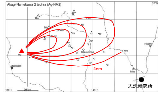
第18図 赤城行川2テフラ(Ag-NM2)の分布 数字は降下火砕堆積物の層厚で、単位はcm。Ag = 赤城火山；Hu = 燧ヶ岳火山；Kn = 鬼怒沼火山；Ni = 男体火山；Tk = 高原火山。
