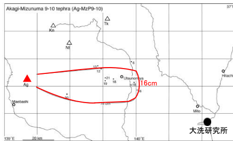
第23図 赤城水沼9-10テフラ(Ag-MzP9-10)の分布 数字は降下火砕堆積物の層厚で、単位はcm。Ag = 赤城火山；Hu = 燧ヶ岳火山；Kn = 鬼怒沼火山；Ni = 男体火山；Tk = 高原火山。
