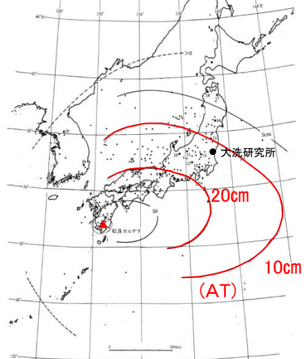
図 2.1-6 始良 Tn 火山灰 (AT) の等層厚線図と主な産出地点。 点線内は入戸大砂流堆積物 (A-Ito) の分布範囲を示す。
