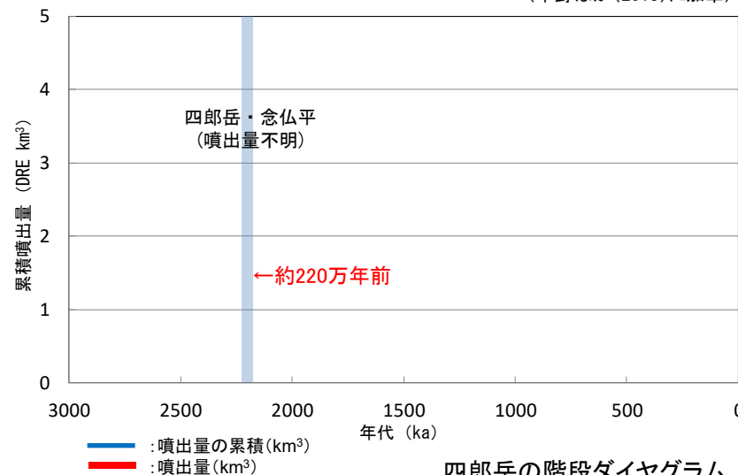
四郎岳の階段ダイヤグラム
