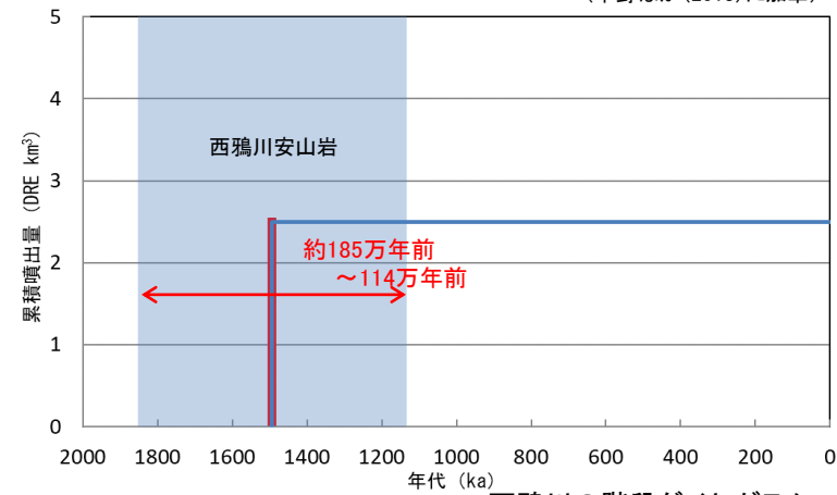
— : 噴出量の累積(km 3 ) — : 噴出量(km 3 ) 西鴉川の階段ダイアグラム
