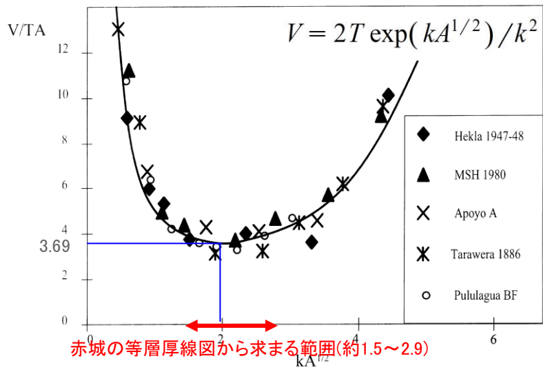
V/TAとkA 1/2 の関係 (Legros(2000)に加筆)
