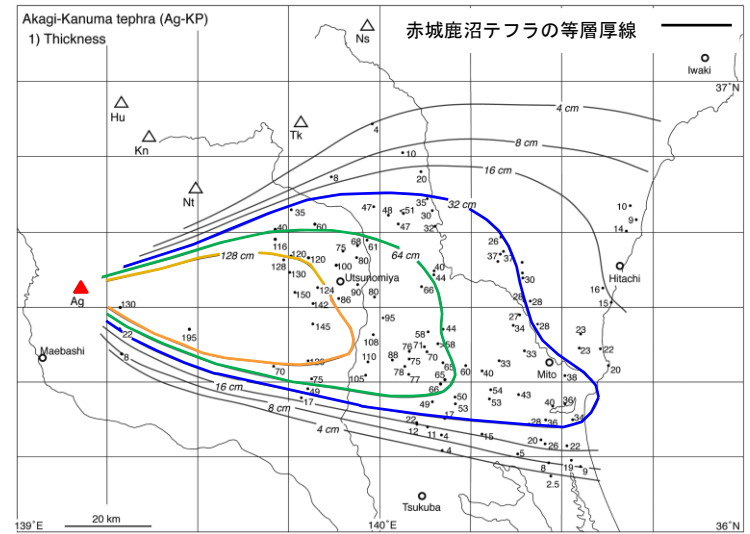
山元(2013a)による赤城鹿沼テフラ(Ag-KP)の分布 (山元(2013a)に加筆)
