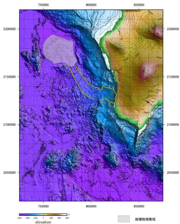
「Alikea-2」の海底地すべり判読結果(現況地形)
