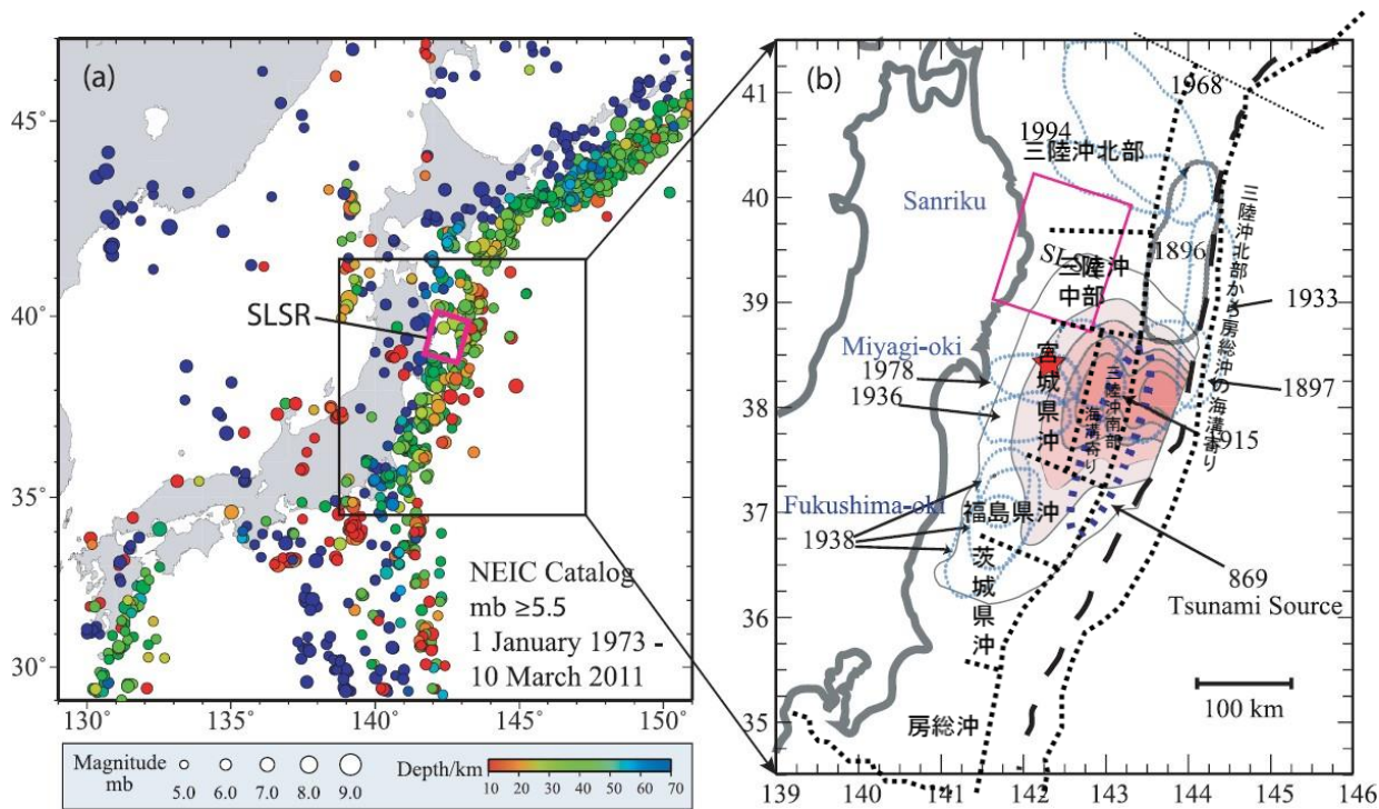
左: 米国立地震情報センター(NEIC)による1973年から2011年東北地方太平洋沖地震以前のM5.5以上の地震の震源分布 右: SLSRの位置(赤線), 主要既往地震の震源域(水色線), 1896年明治三陸地震の波源域(灰色線), 及び東北地方太平洋沖地震のすべり量分布のコンター 三陸沖中部における低地震活動領域(SLSR)と地震の分布の関係
