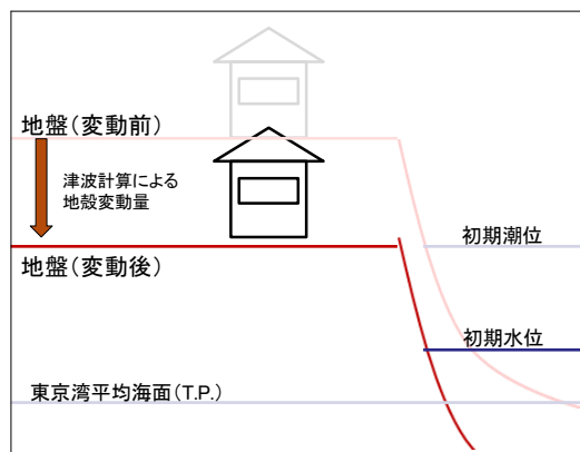
津波計算開始時
