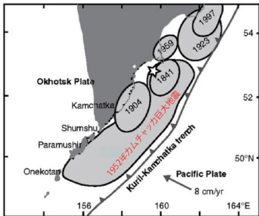
図2 カムチャッカ沖で発生した最近の巨大地震の震源域 (Fedotov et al., 1982) . ☆は 1952 年カムチャッカ巨大地震の震源を示す. MaclInnes et al.(2010)の図に追記した.
