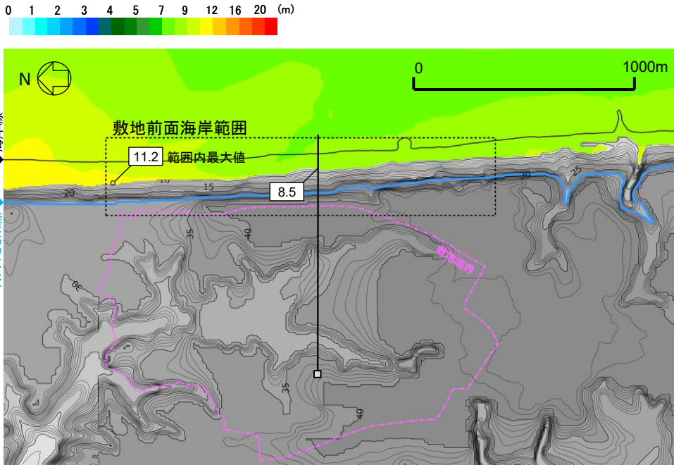
津波高さ分布図(位置:基準)
