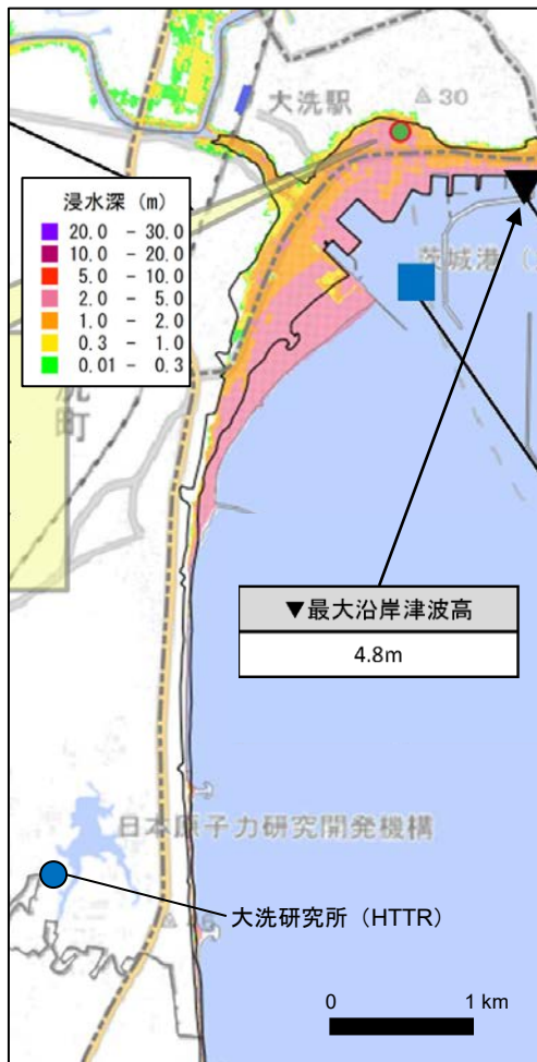
日本海溝・千島海溝沿いの最大クラスの津波による浸水想定 （内閣府（2020, 2022） 一部加筆）
