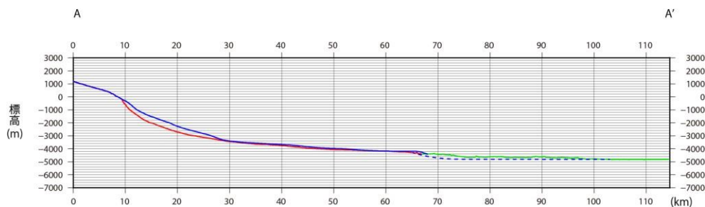
「Alikea-2」の海底地すべり判読結果(現況地形)
