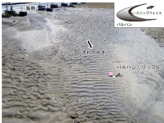
図5 図. 道路の分離帯に形成されたリップルを持つ津波堆積物 (2011/3/13)。海岸から400m付近の遡上流による堆積物。淘汰の良い細粒砂層からなり、層厚は最大で約10cm。リップルの波長は長いもので10cm。写真中央には直線状のカレントリップル、左手には舌状のカレントリップル、右手には三日月形のパルハンが見られる。活断層・地震センターのHPより転載。
