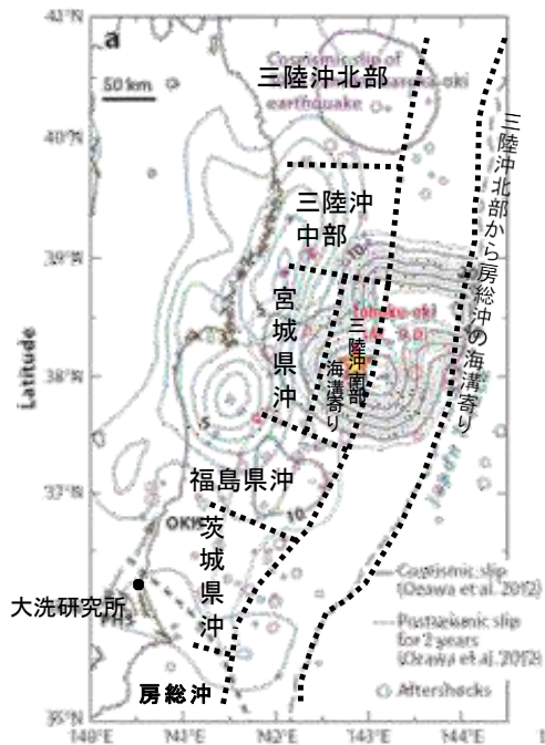
陸上・海上のGPS及び水圧計データに基づく2011年東北地方太平洋沖地震のすべり量分布(黒線) (Ozawa et al. (2012)に加筆)
