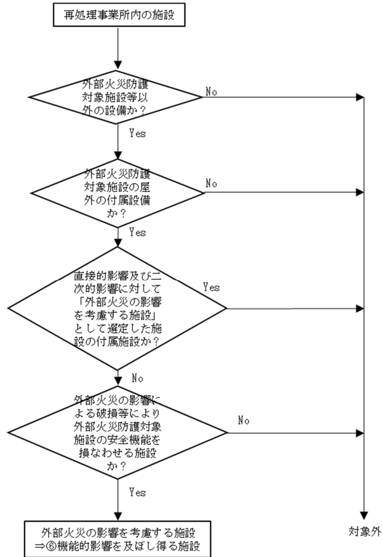
第 2-4 図 機能的影響を及ぼし得る施設の選定フロー
