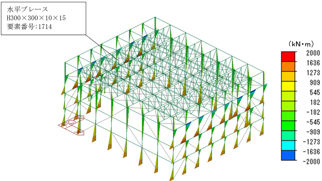
第4-18図 曲げモーメント図 (Mz) (ケース1-1)
