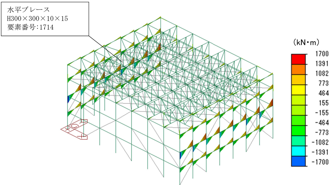
第4-17図 曲げモーメント図 (My) (ケース1-1)
