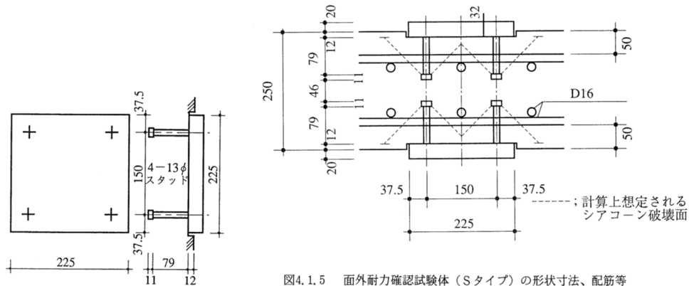
図4.1.5 面外耐力確認試験体（Sタイプ）の形状寸法、配筋等
