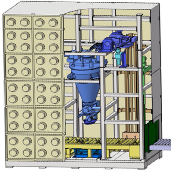
第 4.3-4 図 グローブボックス概要図
