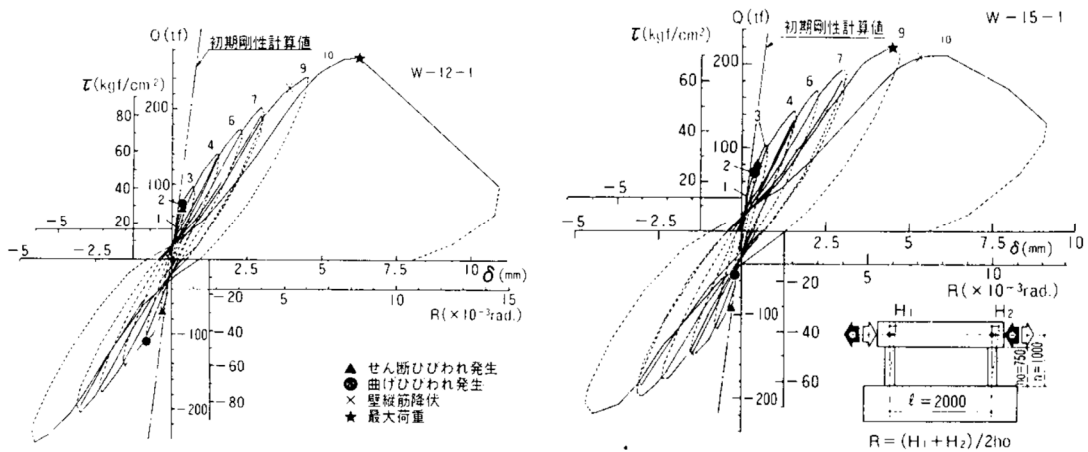
(c) 荷重-変形関係
