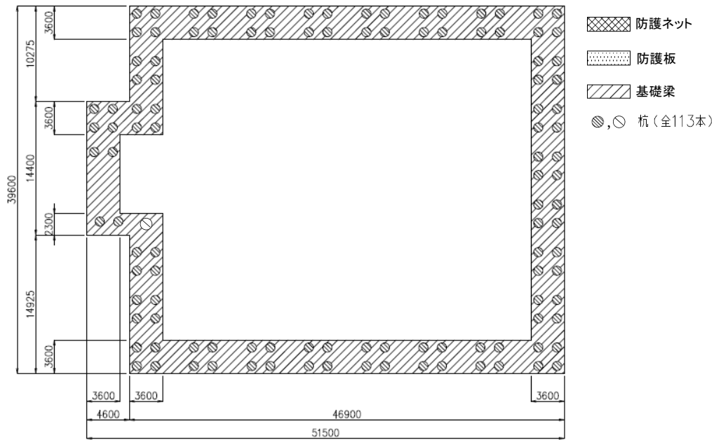
(杭伏図)
