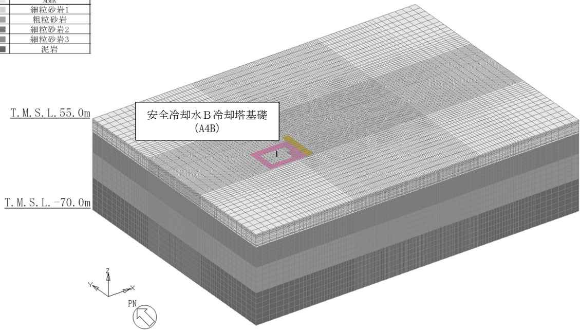
(a) 全体図
