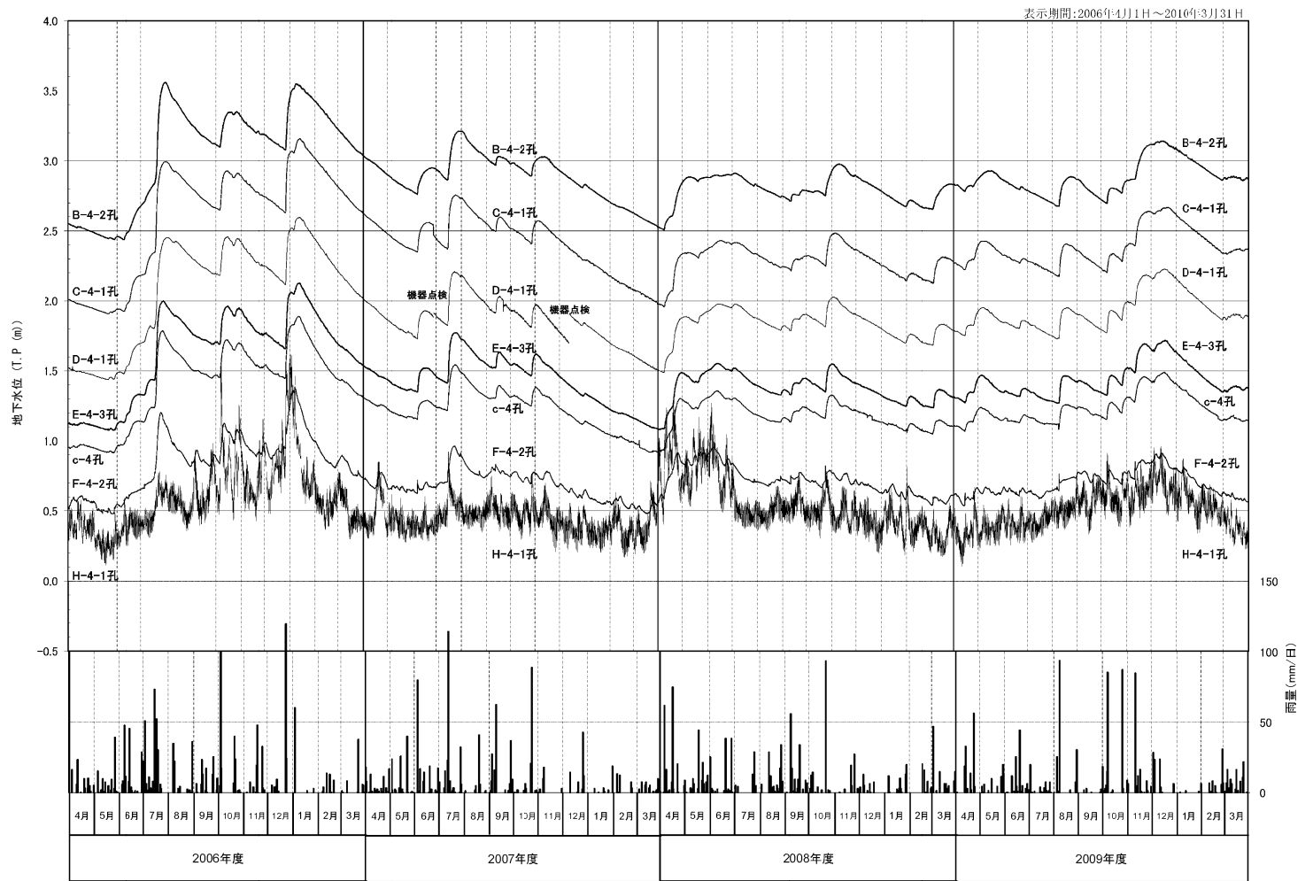
第 1.6.2-6 図 (1) 地下水位観測結果
