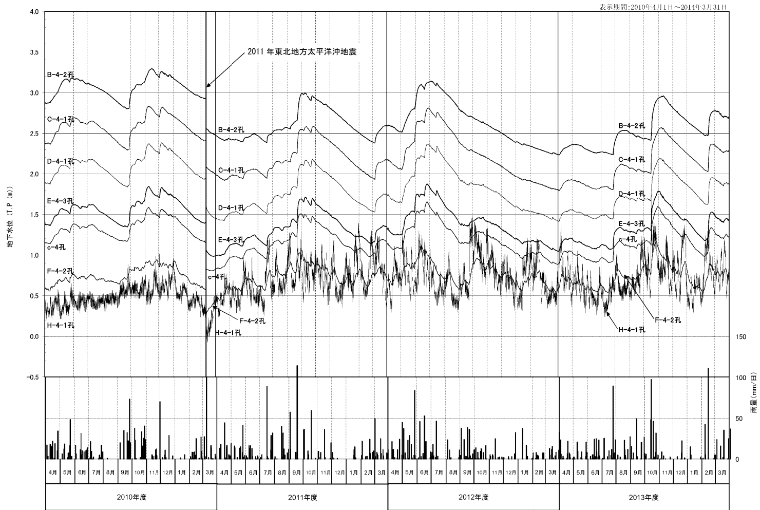
第 1.6.2-6 図 (2) 地下水位観測結果
