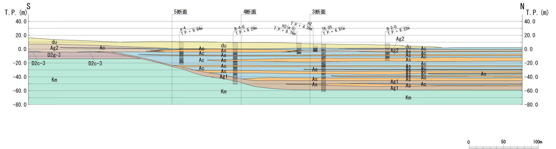
第 1.5-1 図 (4) 廃棄物埋施設位置付近の地質断面図 (B 断面)
