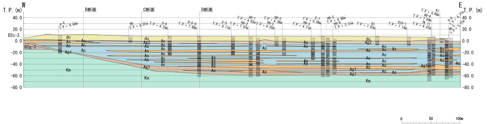
第 1.5-1 図 (3) 廃棄物埋設施設位置付近の地質断面図 (5 断面)
