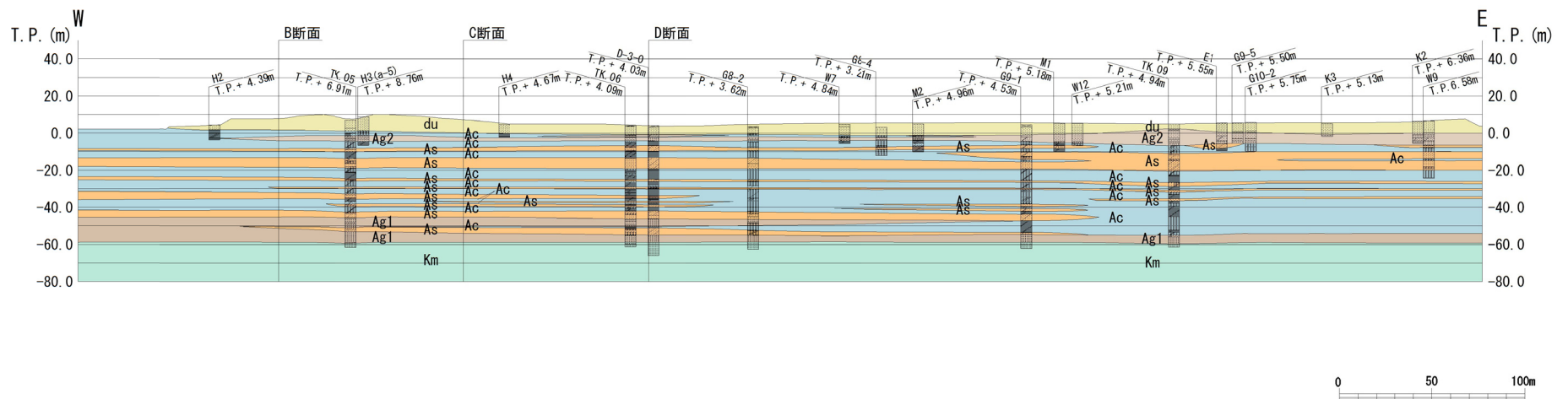
第 1.5-1 図 (1) 廃棄物埋施設位置付近の地質断面図 (3 断面)
