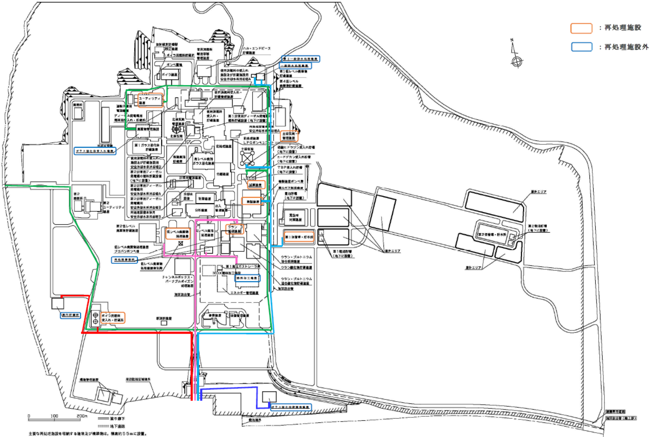
第5図 有毒ガスの発生源となる敷地内可動源を受け入れる建屋の配置及び輸送ルート(例)
