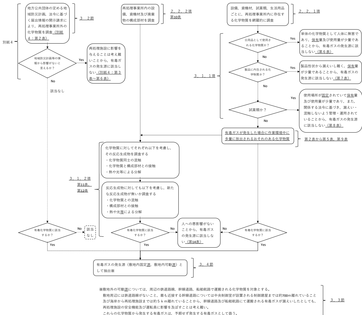
第1図 有毒ガスの発生源の抽出フロー
