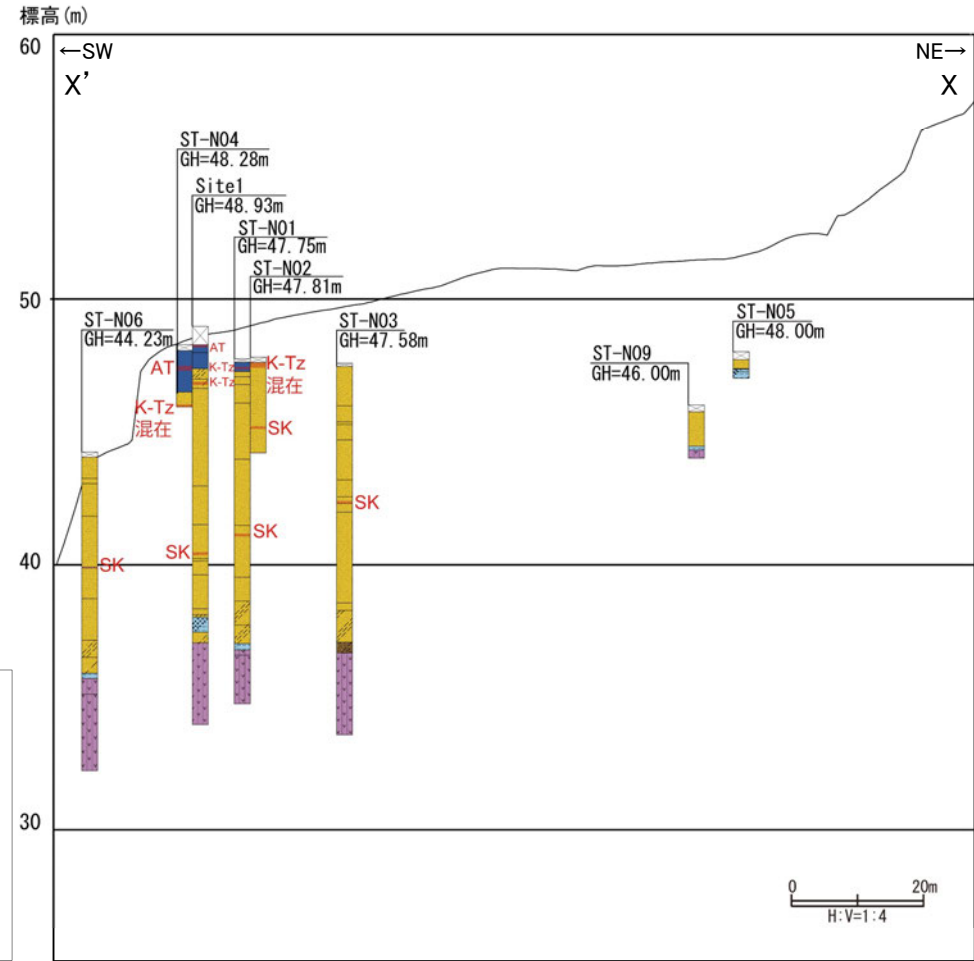
断面図
