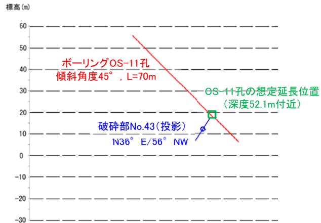
断面図
