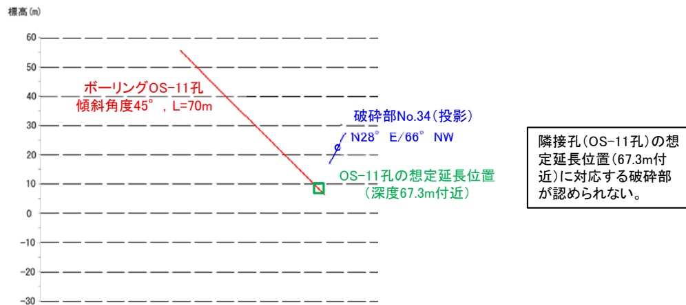
断面図
