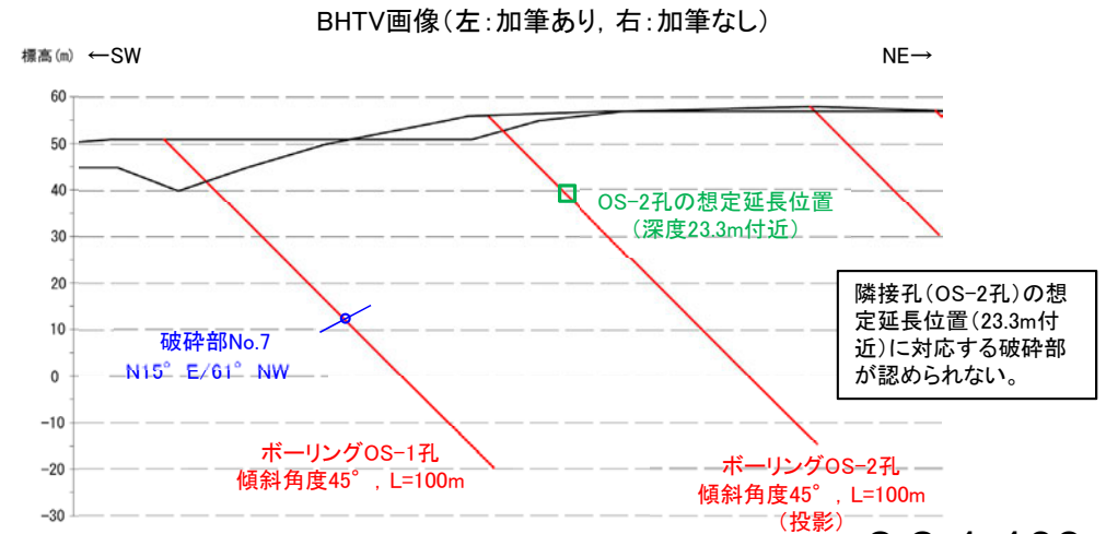
断面図
