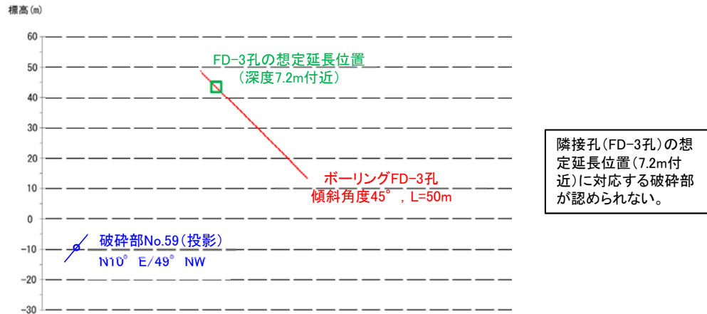
断面図
