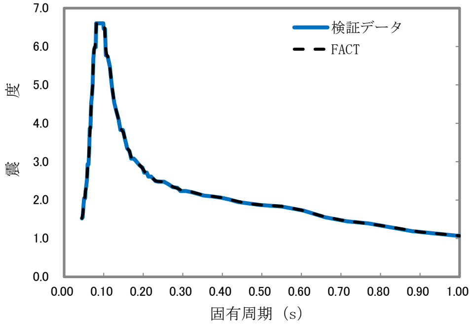
図 3-3 検証用データと本解析コードの比較結果 (EW 方向床レベル 55.30m 減衰 1.0%)
