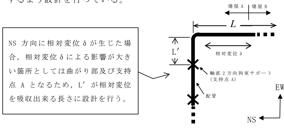
第 2.2.3-1 図 二次応力を考慮した配管設計のイメージ (平面)
