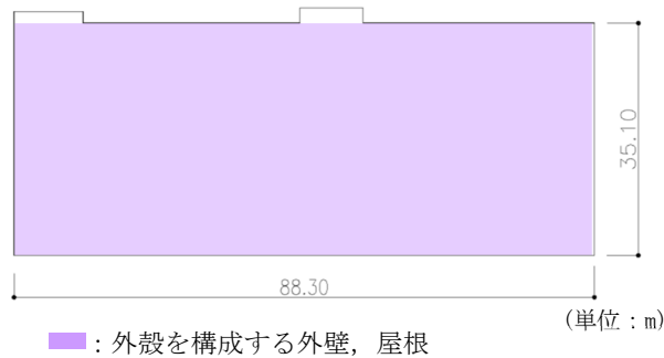
第 5-4 図 概略平面図 (T. M. S. L. 77. 50m)
