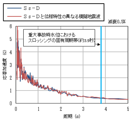
図 3-4 床応答加速度スペクトル
