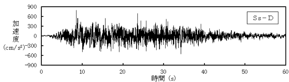
図 3-1 S s - D の応答加速度時刻歴波形
