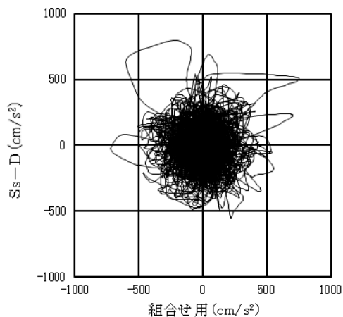
図 3-3 S s - D による建物応答加速度のオービット (位相が異なる地震波を 2 方向入力した場合)
