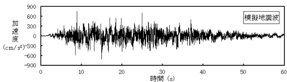
図 3-2 S s - D と位相特性の異なる模擬地震波の応答加速度時刻歴波形
