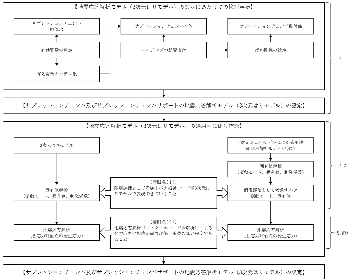
図 4.2-1 3次元はりモデル設定及び適用性検証フロー
