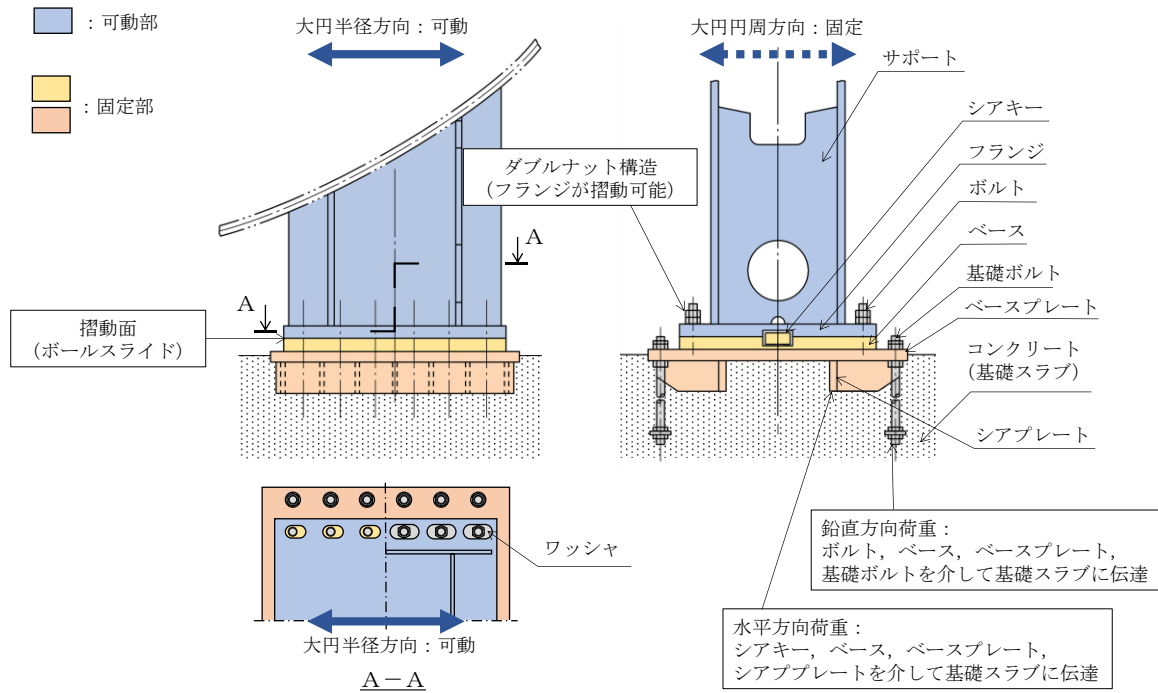
図 2.1-2 サプレッションチェンバサポート構造詳細図
