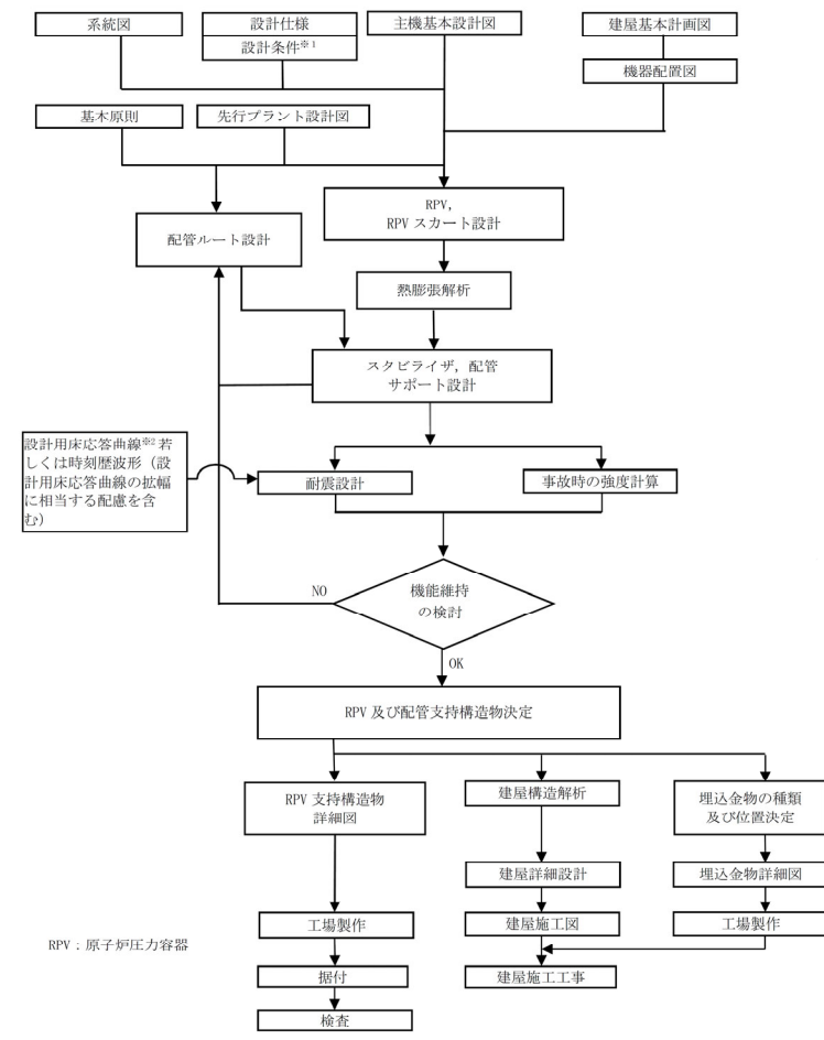
図2-1 主要機器支持構造物設計フロー
