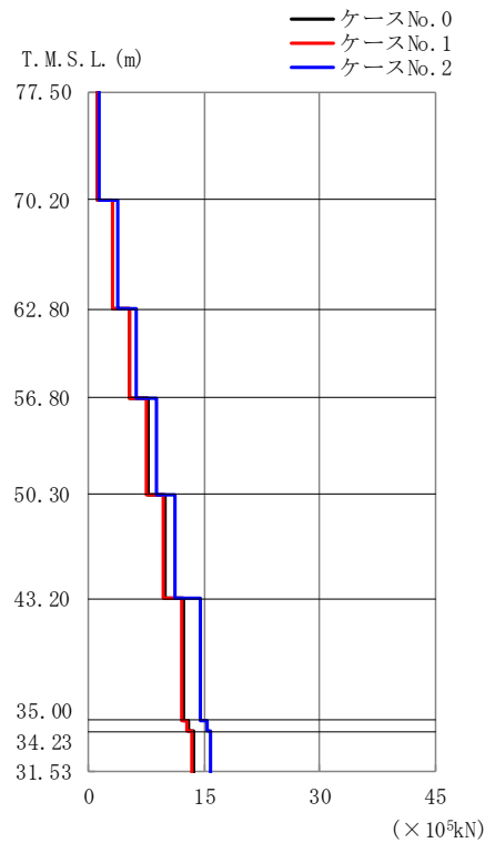
第 4. 1. 3-34 図 最大応答せん断力 (EW 方向) (4/4)
