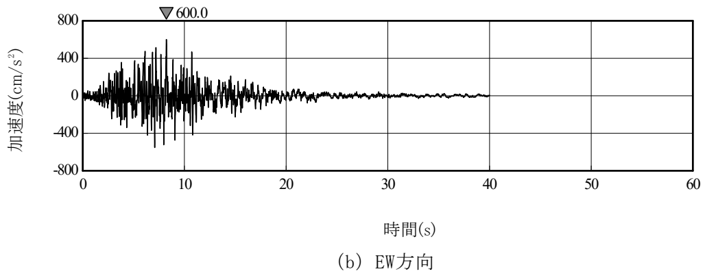
第 4-2 図(10) 1.2×S s -C 4 の加速度時刻歴波形 (燃料加工建屋)
