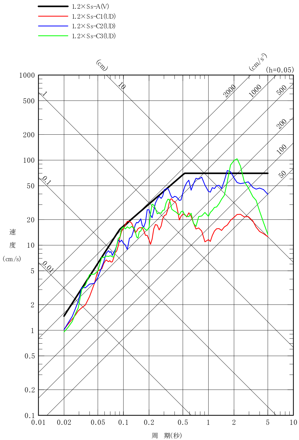
第 4-1 図(5) 1.2×S s - C の応答スペクトル (鉛直方向) (燃料加工建屋)
