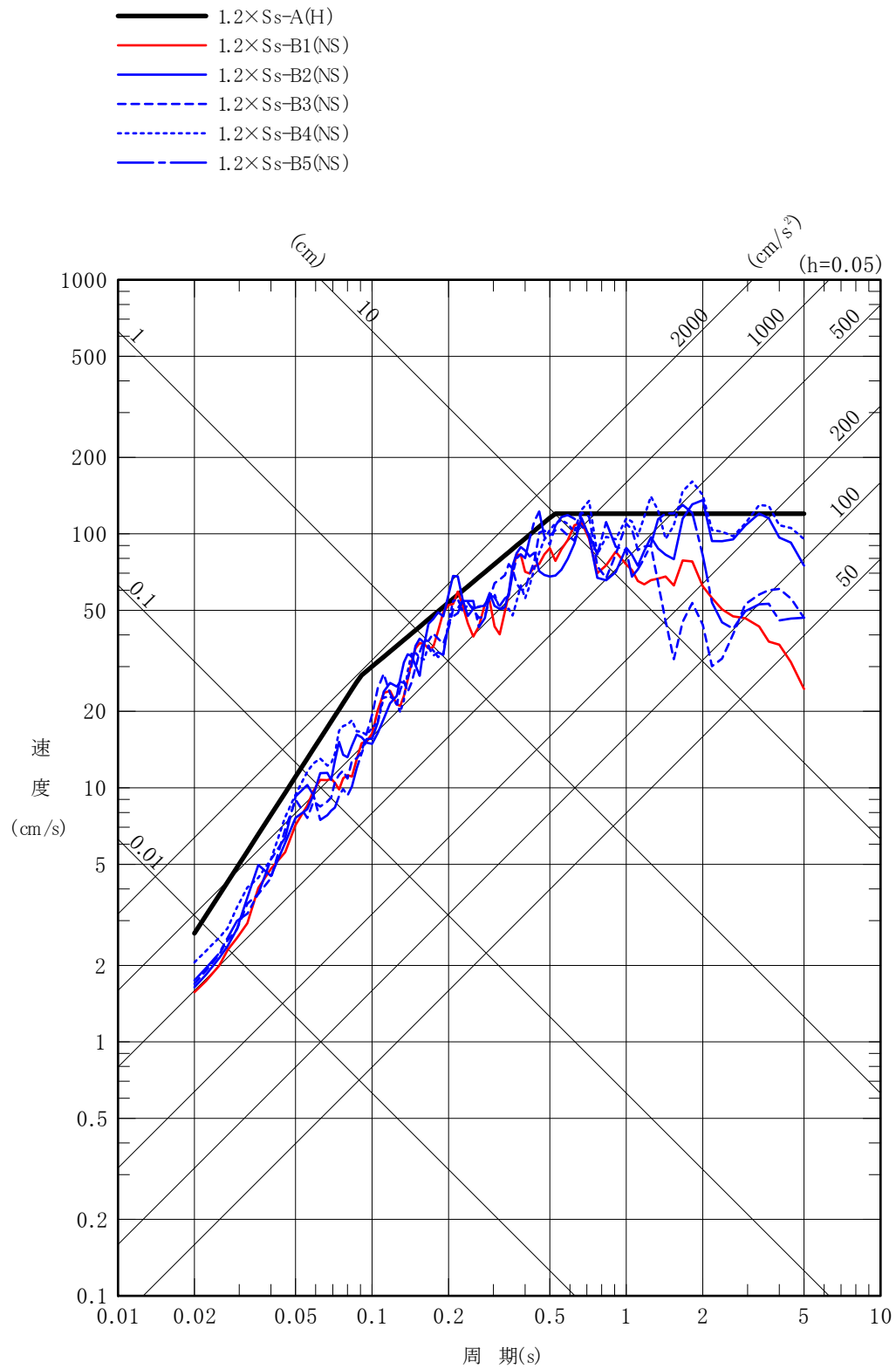
第 4-1 図(1) 1.2×S s -A と 1.2×S s -B の応答スペクトル (NS 方向) (燃料加工建屋)
