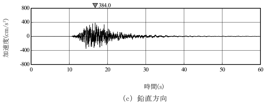
第 4-2 図(8) 1.2×S s -C2 の加速度時刻歴波形 (燃料加工建屋)
