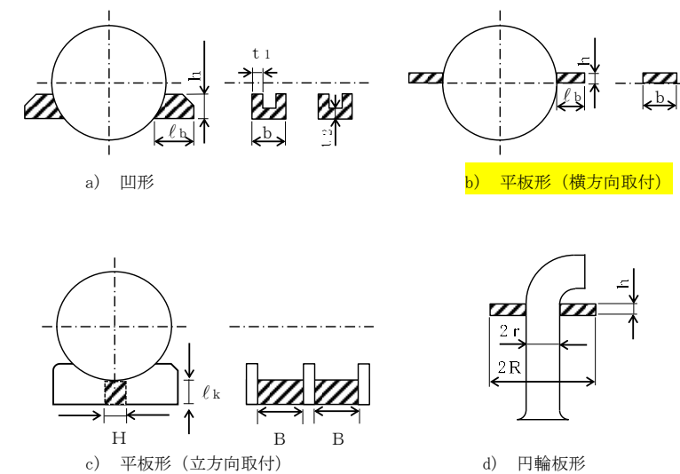
図 2-1 支持構造物の形状例
