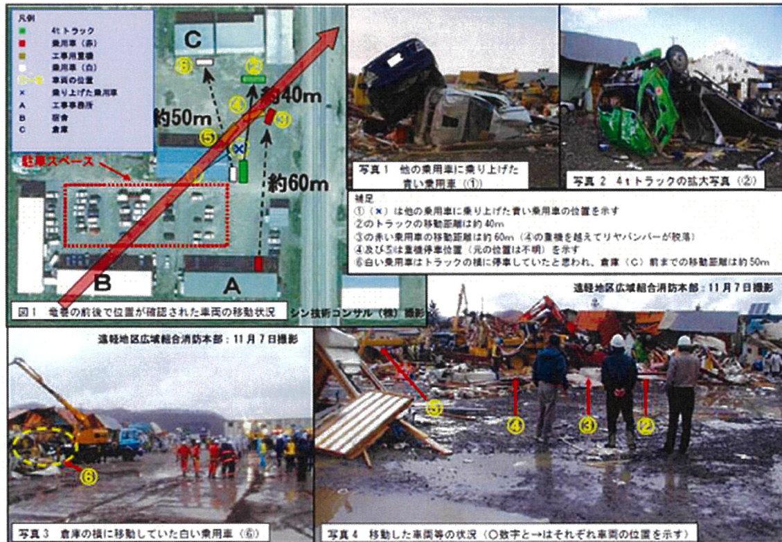
佐呂間竜巻(2006. 11. 7)による被災状況: 工事事務所敷地内の車両被災 (竜巻経路 → を追加)
