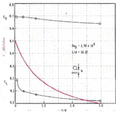
(円柱の場合)
