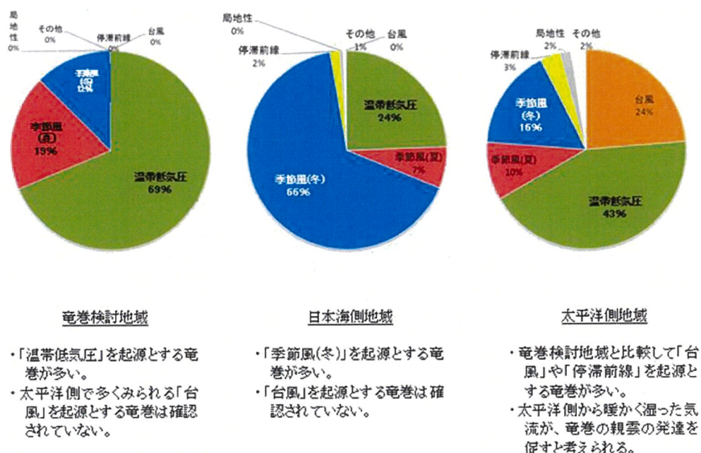
第7図 竜巻の総観場の特徴の比較
