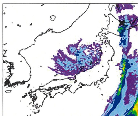
別添 2-2 図 2006/11/07 F3 事例における環境場と突風関連指数 (左) 500 m 高度における風向・風速および相当温位 (単位: K) (左下) SReH, (右下) 最大 CAPE
