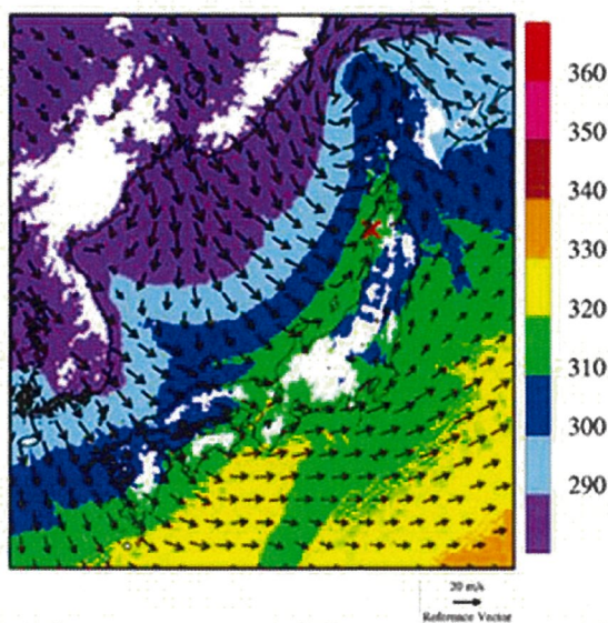
別添 2-10 図 1999/11/25 F1-F2 事例における環境場と突風関連指数(左) 500 m 高度における風向・風速および相当温位(単位: K) (左下) SReH, (右下) 最大 CAPE
