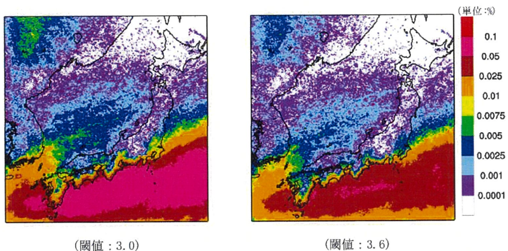
第 24 図 EHI の超過頻度分布 (閾値 : 3.0, 3.6)
