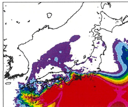
別添 2-3 図 1999/09/24 F3 事例における環境場と突風関連指数 (左) 500 m 高度における風向・風速および相当温位 (単位: K) (左下) SReH, (右下) 最大 CAPE
