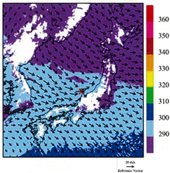
別添 2-8 図 1990/04/06 F2 事例における環境場と突風関連指数 (左) 500 m 高度における風向・風速および相当温位 (単位: K)
