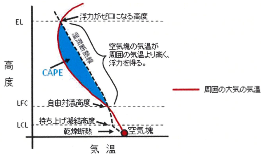
第 17 図 CAPE の算出概念
