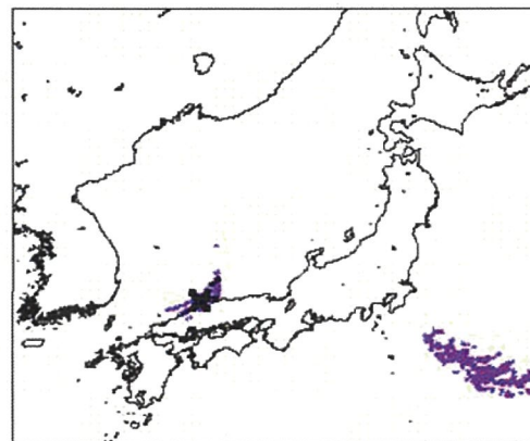
別添 2-9 図 1989/03/16 F2 事例における環境場と突風関連指数 (左) 500 m 高度における風向・風速および相当温位 (単位: K) (左下) SReH, (右下) 最大 CAPE
