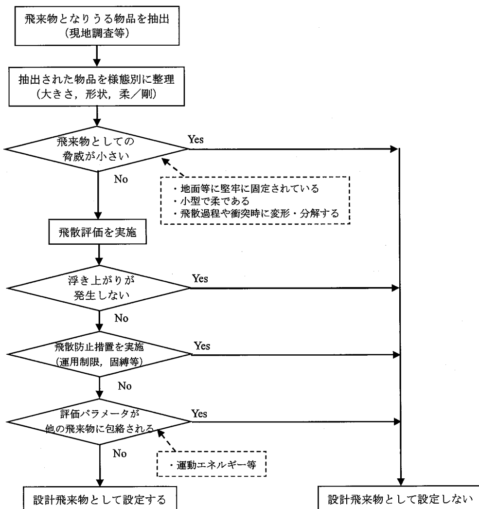
第 43 図 設計飛来物の設定フロー
