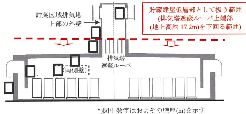
別添5-1図 貯蔵区域断面図(東西方向)
