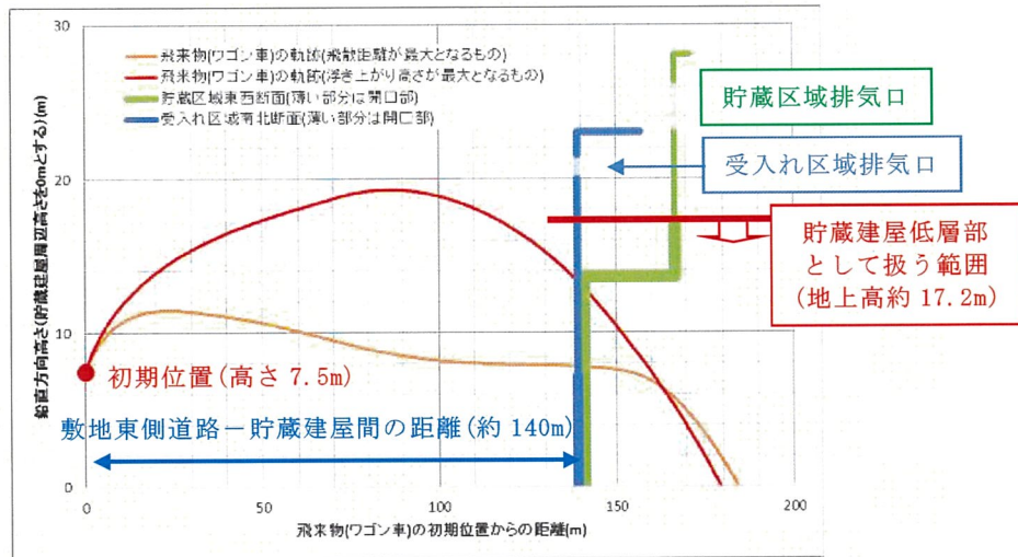
第 48 図 ワゴン車の飛散挙動
