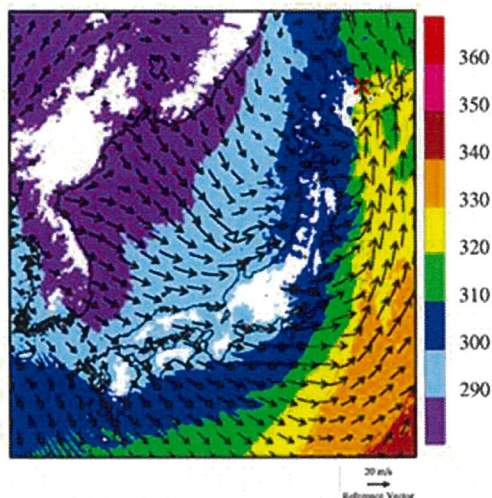
別添 2-2 図 2006/11/07 F3 事例における環境場と突風関連指数 (左) 500 m 高度における風向・風速および相当温位 (単位: K) (左下) SReH, (右下) 最大 CAPE
