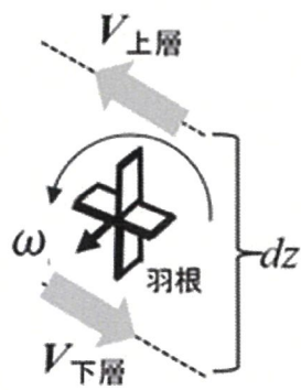
水平渦度生成に関する模式図
