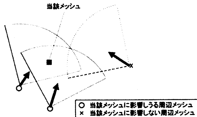
第18図 最大CAPE値の算出方法概念図
