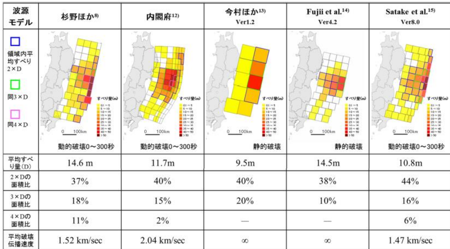
2011年東北地方太平洋沖地震のすべり分布及び断層破壊モードの分析結果
