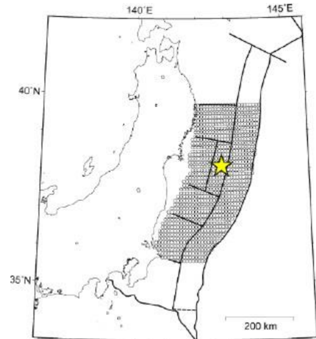
確率論的地震動予測地図の作成に用いた「東北地方太平洋沖型の地震」の断面図(地震調査研究推進本部(2014))
