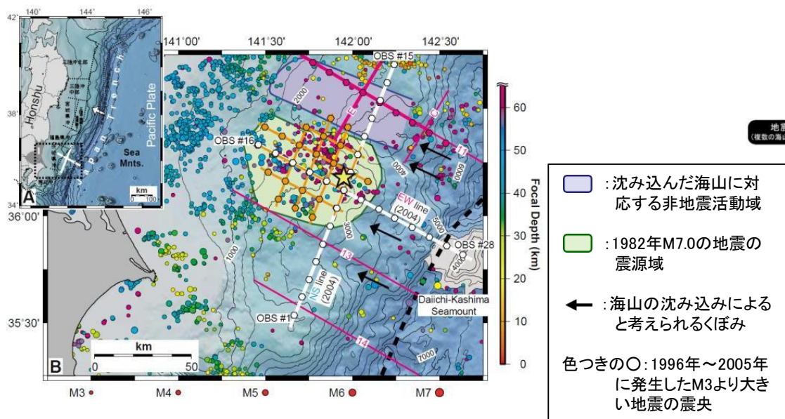
複数の海山が沈み込んだ領域と地形及び地震活動の関係 (Mochizuki et al. (2008)に加筆)
