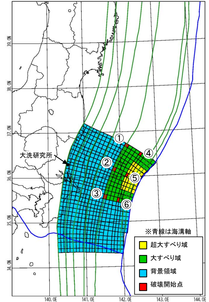
破壊開始点位置図
