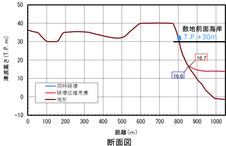
断面図
