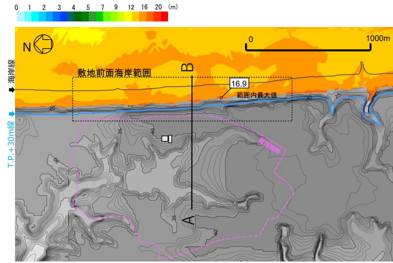
(プレート間地震: 茨城県沖から房総沖に想定する津波波源)
